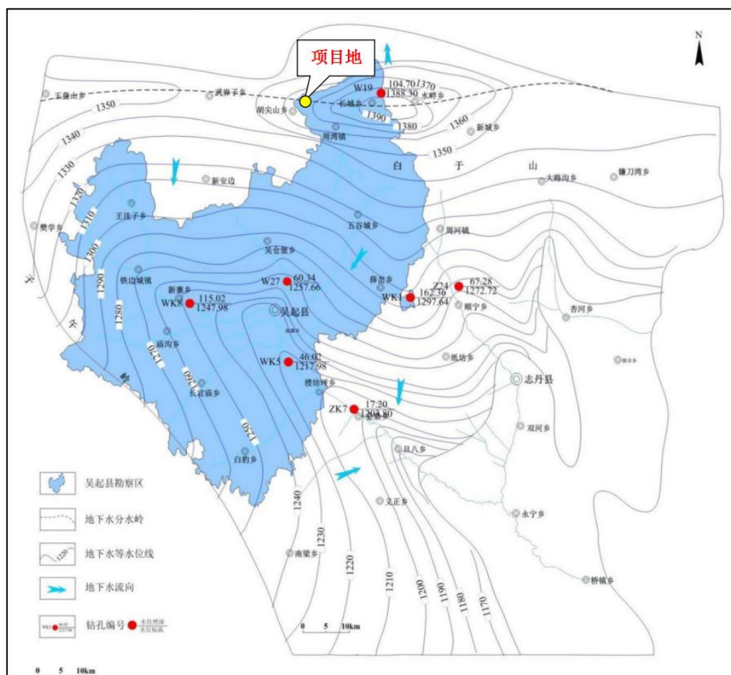
图 4.1.4-4 白垩系环河组地下水水流场图
