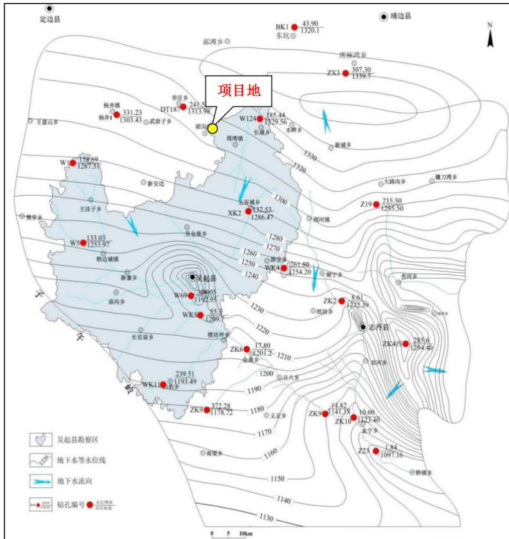
图 4.1.4-5 白垩系洛河组地下水流场图
