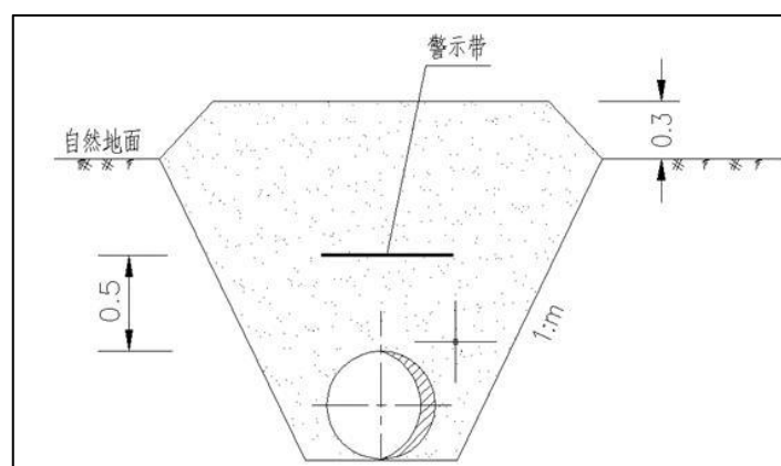
图 2.4.2-2 管沟断面示意图
