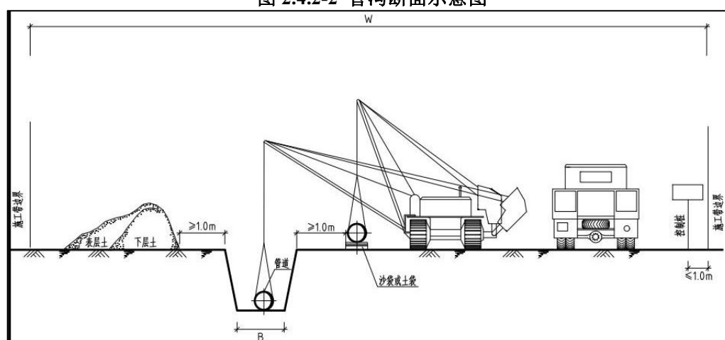
图 2.4.2-3 管沟开挖施工工艺示意图
