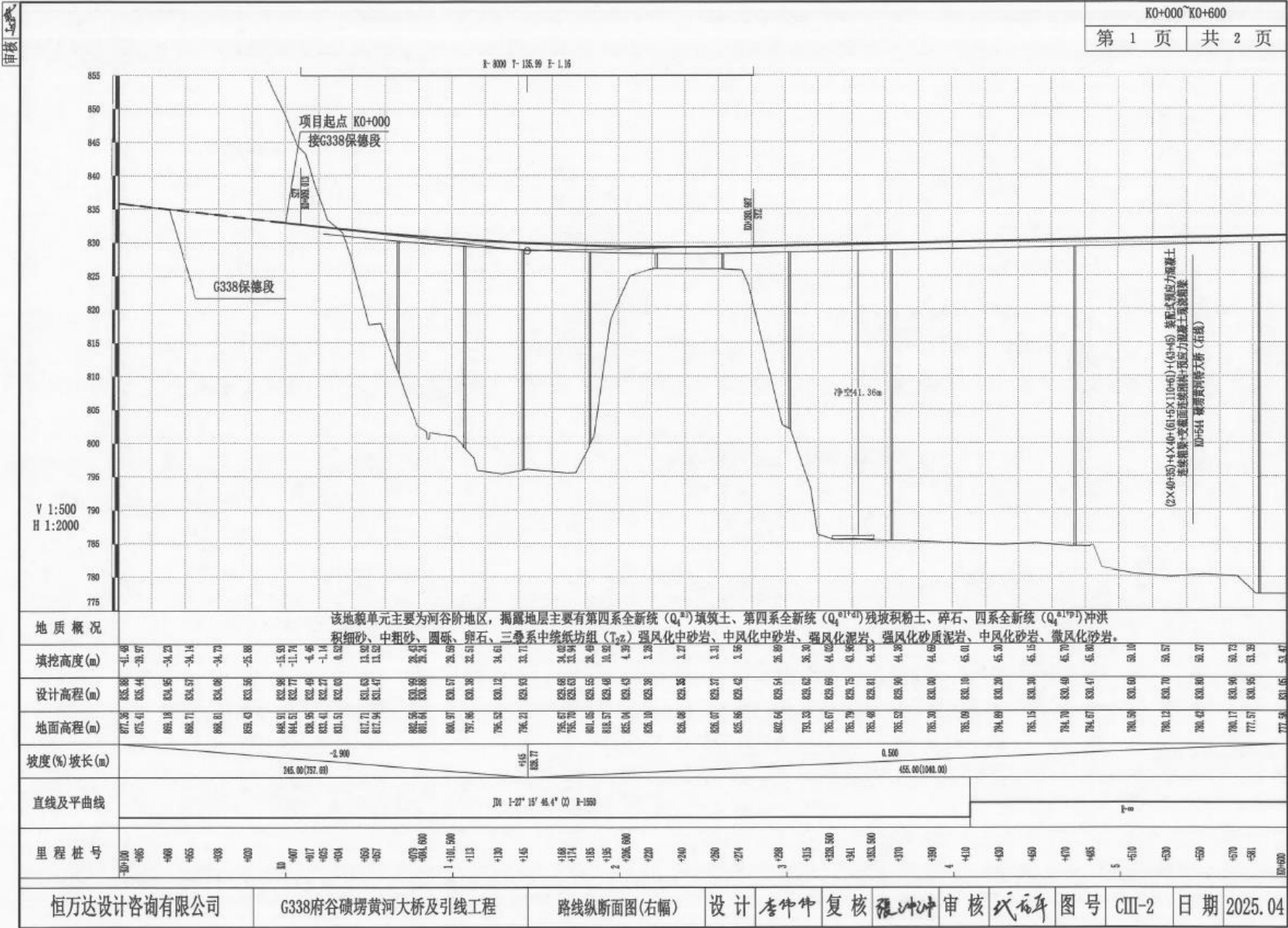
图 2.5-15 项目路线纵断面图（右幅）1
