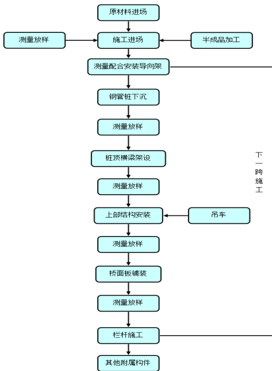
图 3.1-4 施工便桥安装工艺流程图
