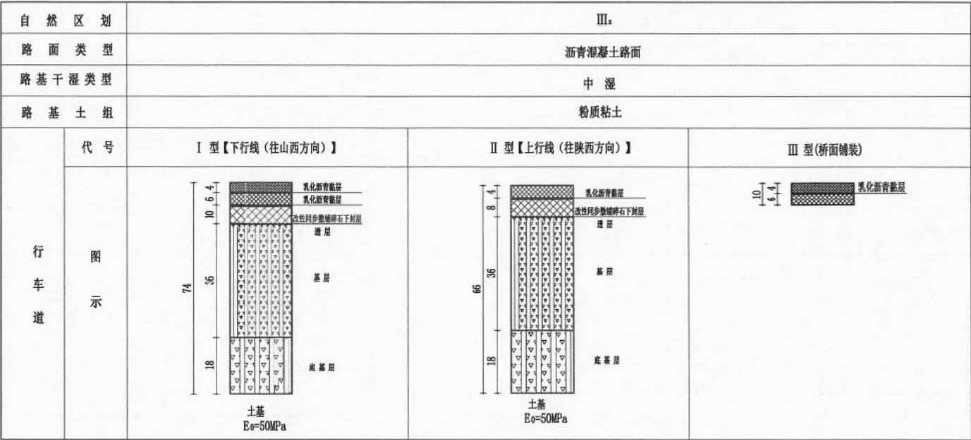
路面结构设计图
