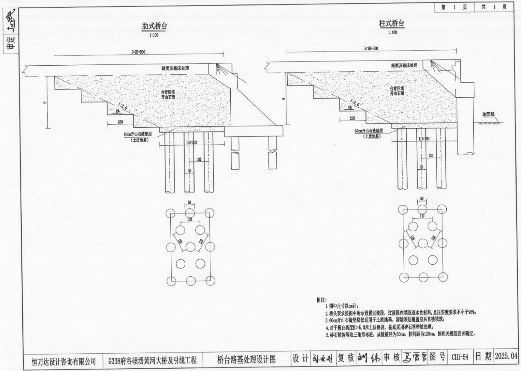
图 2.5-2 桥台路基处理设计图
