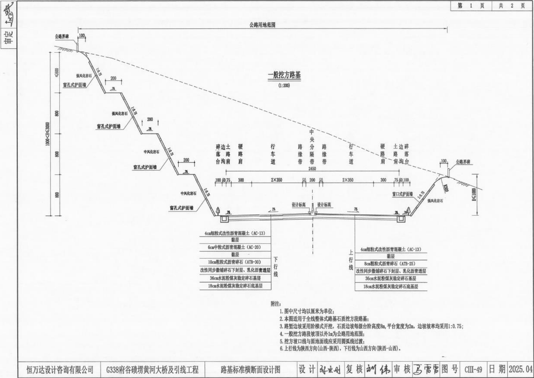
图 2.5-1 整体式路基标准横断面图
