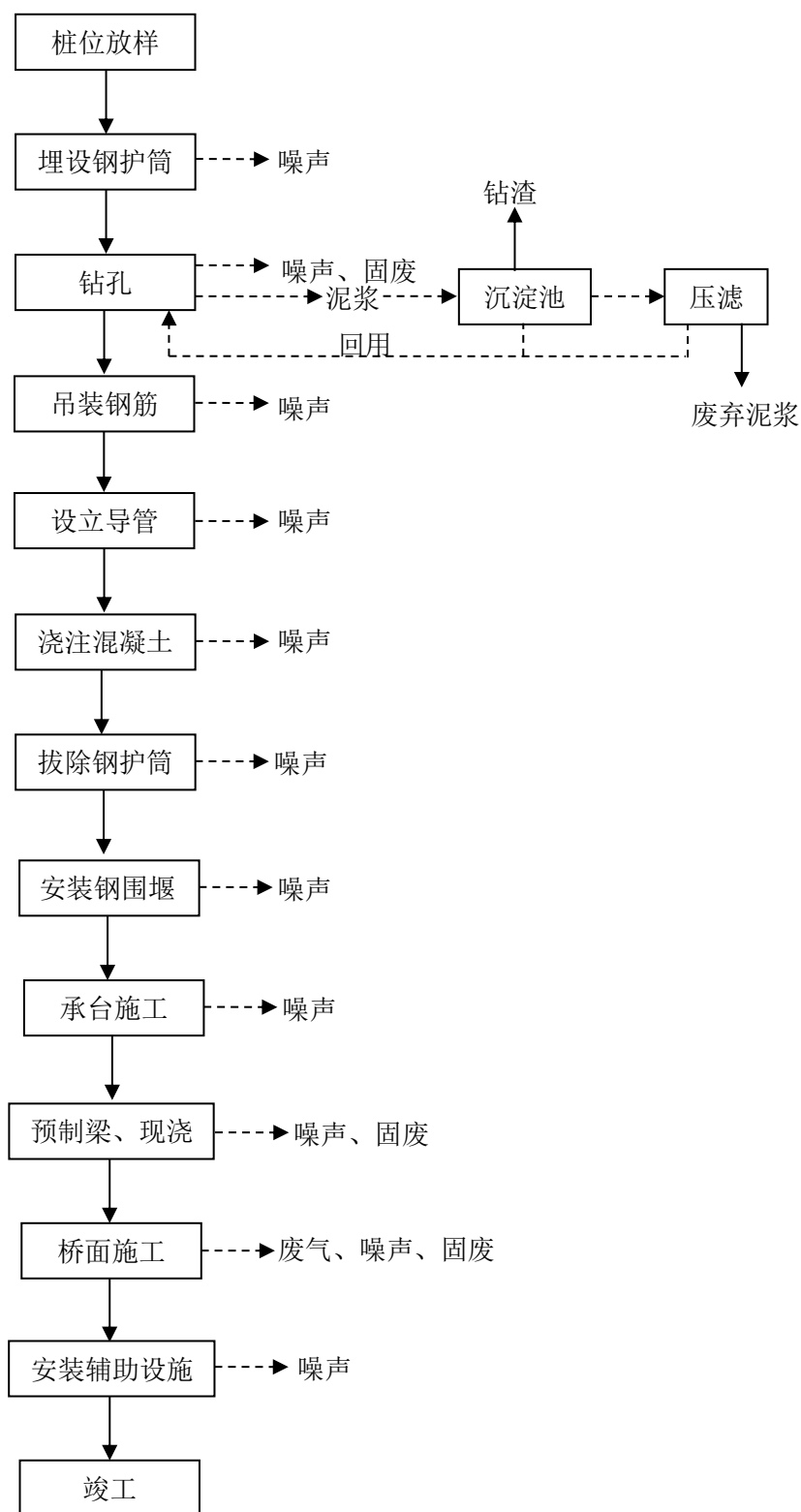
图 3.1-3 桥梁建设工艺流程及产污节点图
