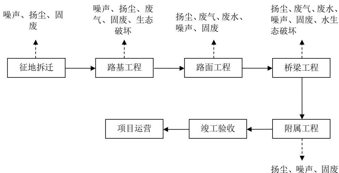
图 3.1-6 项目工艺及产污节点图
