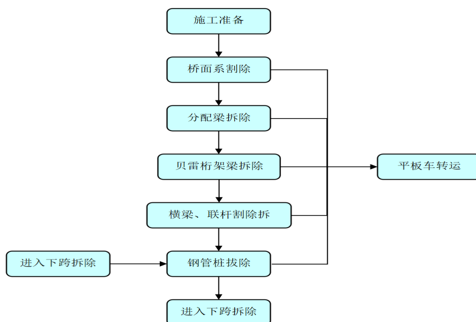
图 3.1-5 施工便桥拆除工艺流程图
