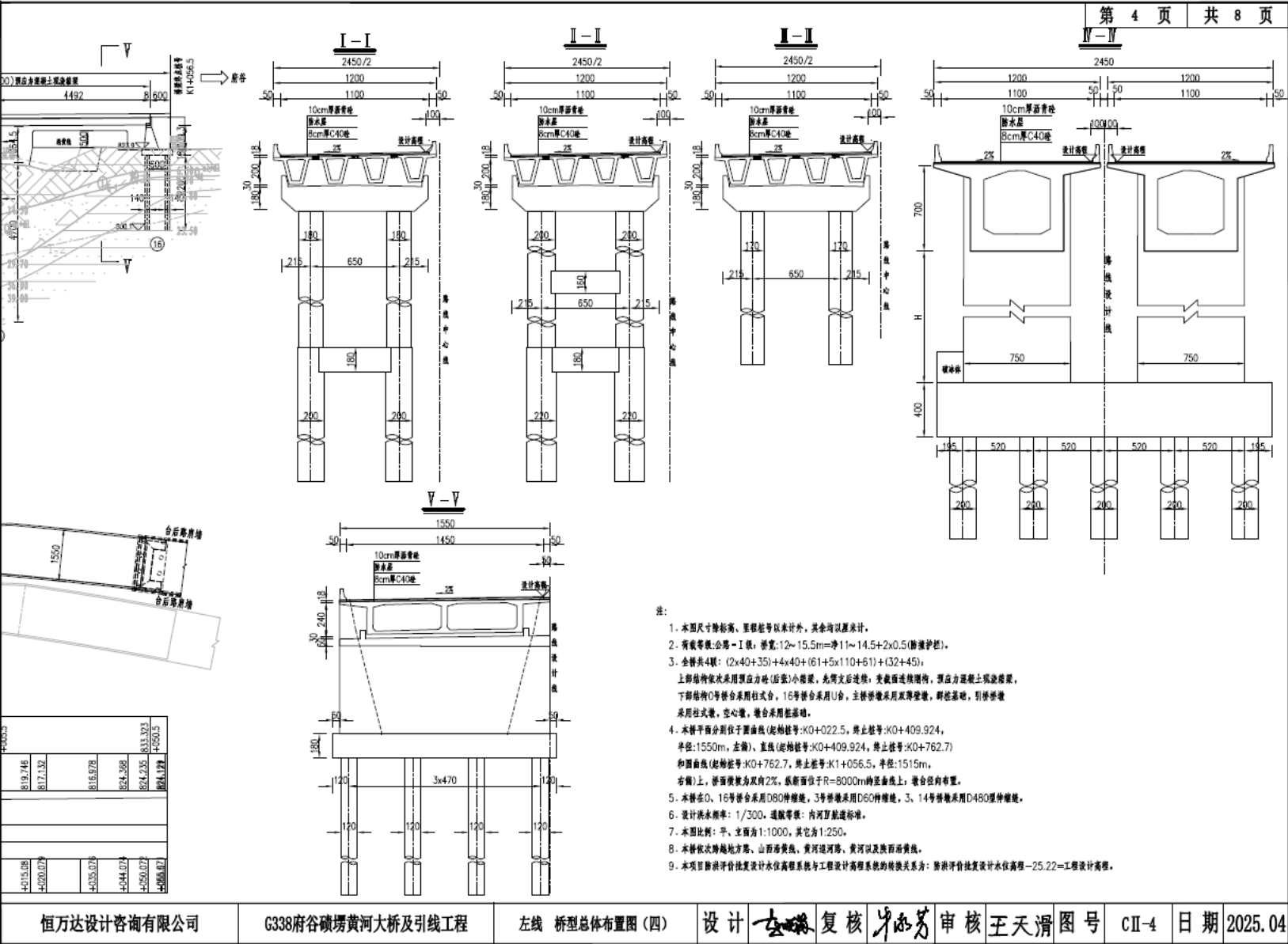
图 2.5-20 桥型总体布置图(左幅) 4
