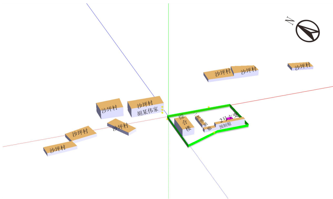
图 4-7 江口 110 千伏变电站噪声仿真预测三维模型图
