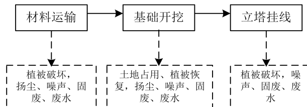
图 4-3 架空线路施工期工艺流程及产污环节示意图
