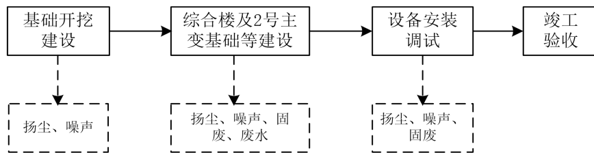
图 4-1 扩建江口 110 千伏变电站施工工艺流程及产污环节示意图
