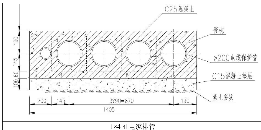
图 2-6 电缆排管剖面示意图
