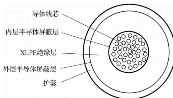
图 3 电缆结构示例图
