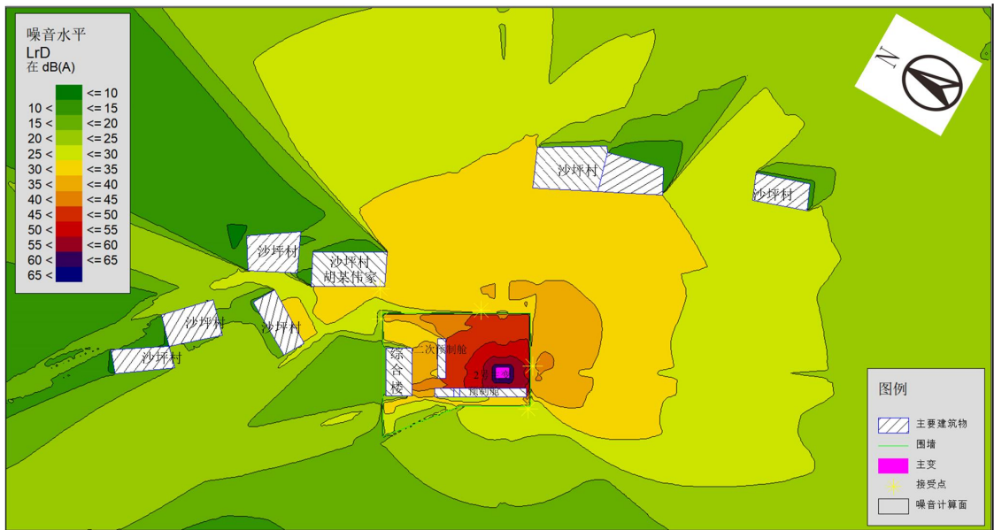
图 4-8 江口 110 千伏变电站等效噪声级预测图
