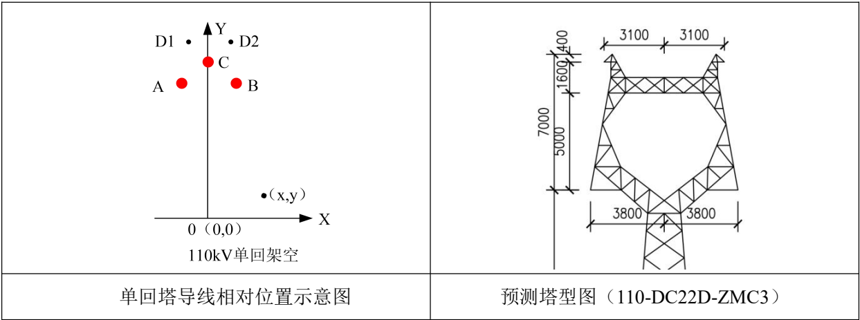
图 4 单回路预测塔型示意图
