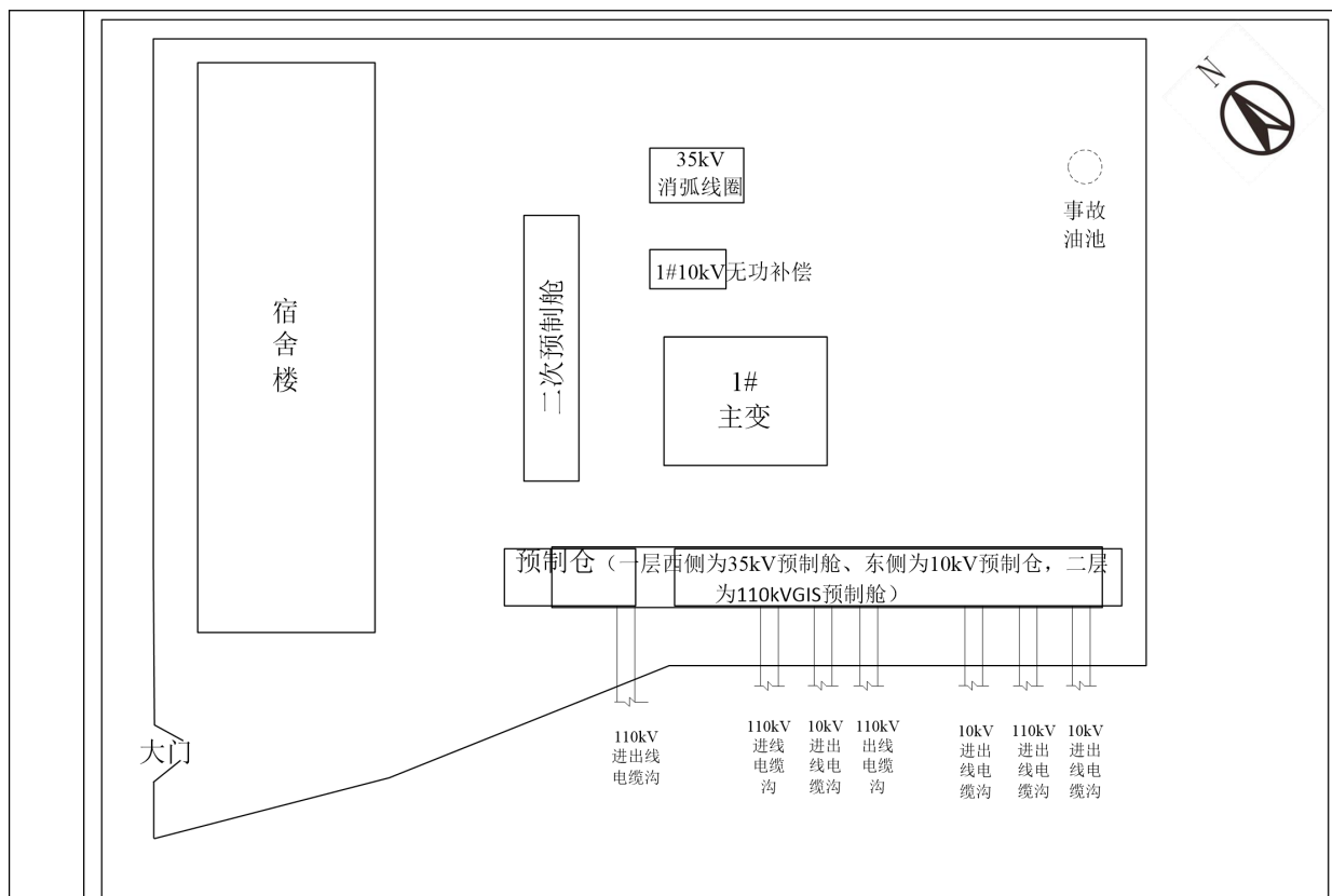
图 2-3 江口 110kV 变电站平面布置示意图（现状）
