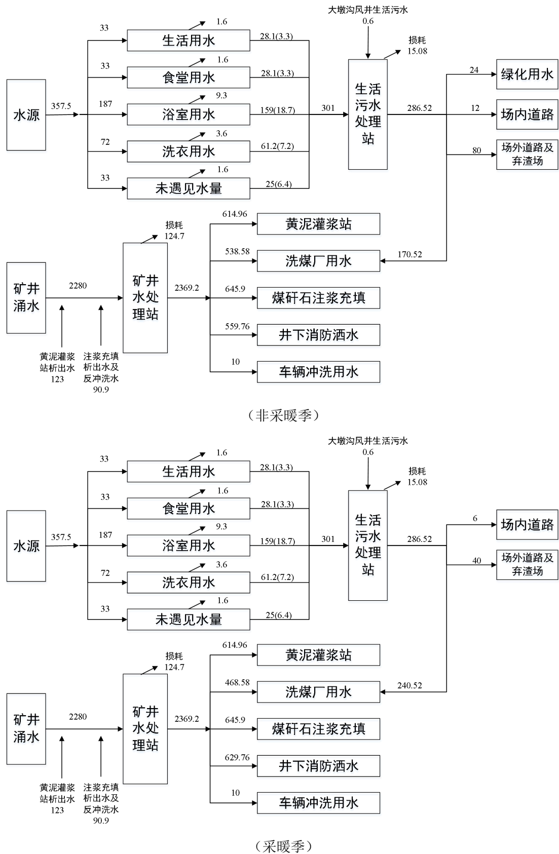
图 2.7.2-2生产能力核定后安山煤矿水平衡图
