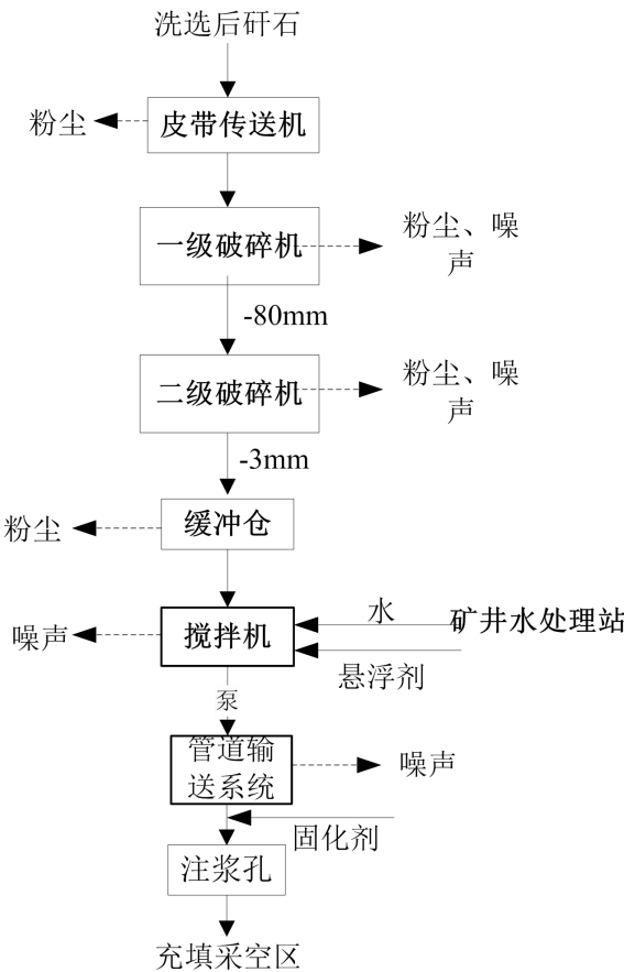
图 2.6.4-3 生产工艺流程及产污环节图
