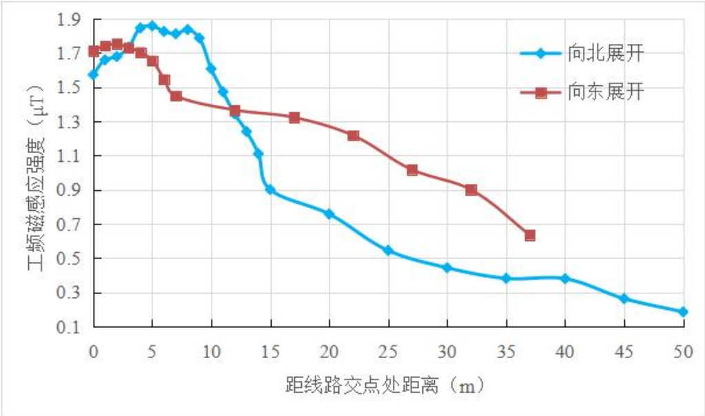
图 6.1-48 330kV 信上 I、II 线跨越 330kV 东咸 I 线断面展开工频磁感应强度变化趋势图
