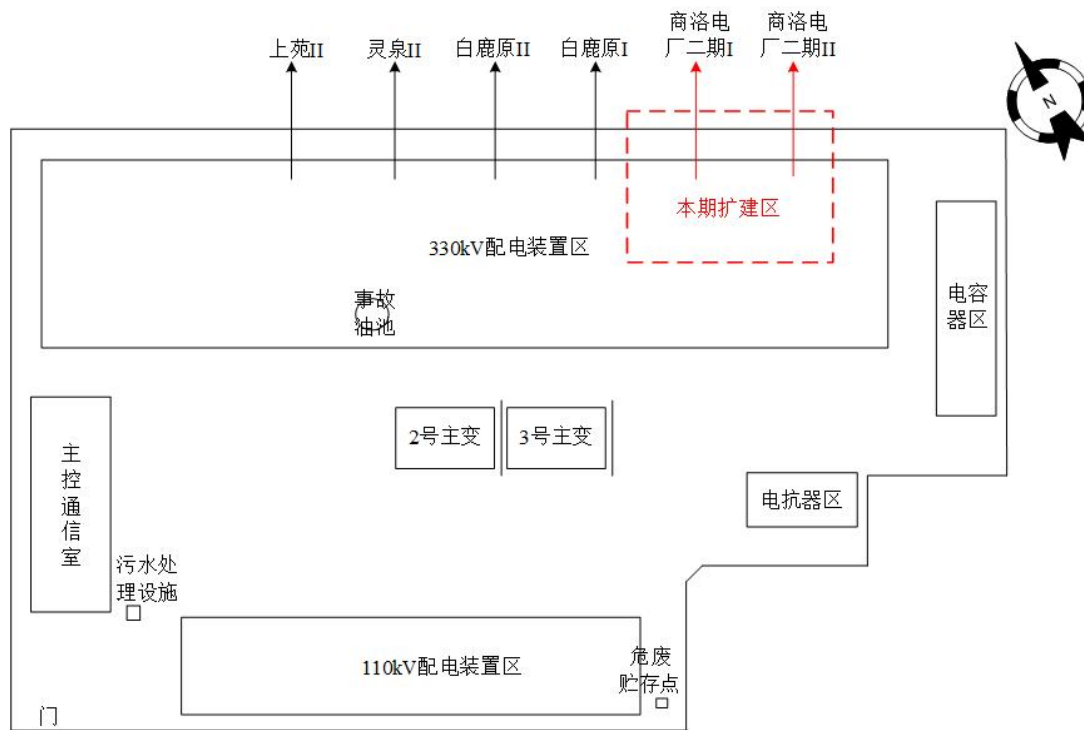
图 3.1-1 美玉 330kV 变电站平面布置示意图
