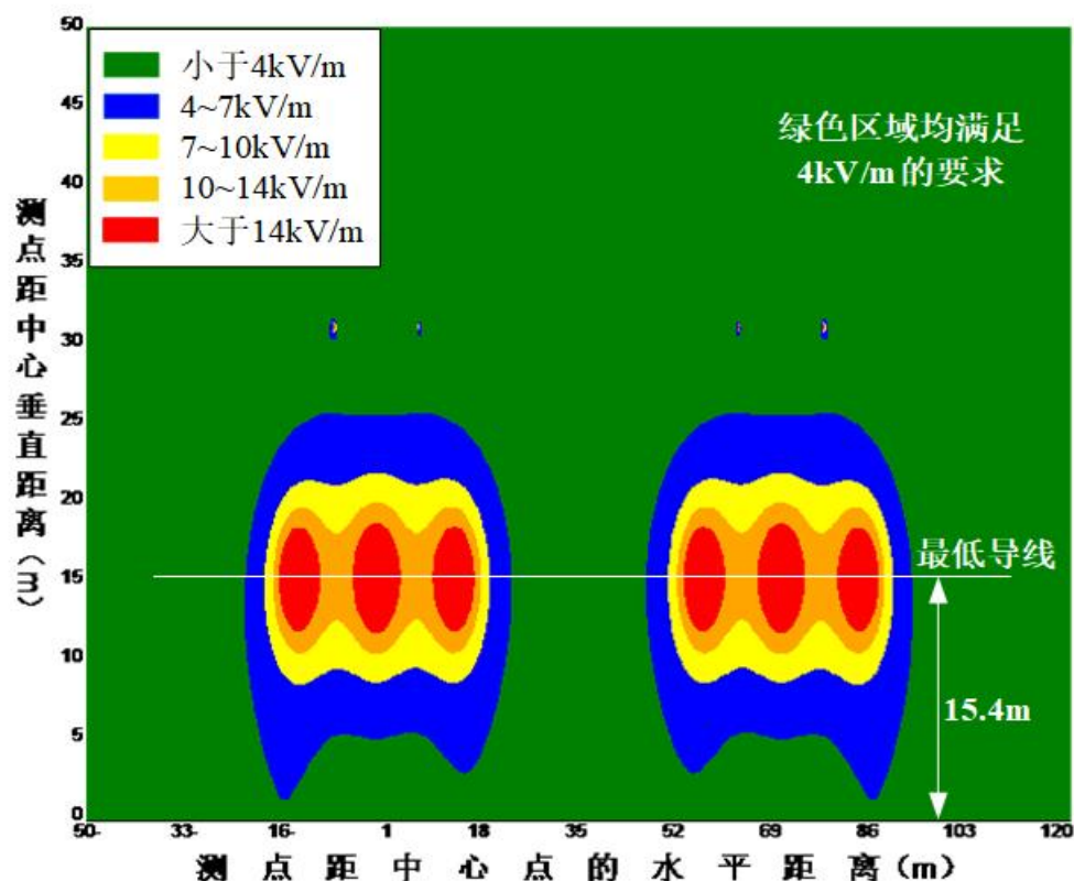
图 6.1-33 本项目单回路工频电场强度空间分布图 (JL3/G1A-400/50-ZBC27202)
