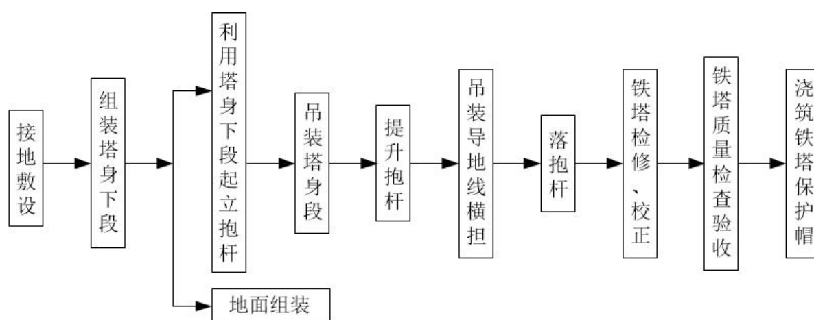
图 3.1-3 铁塔组立施工工艺流程图
