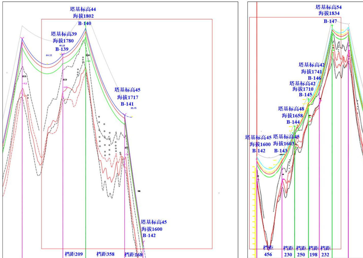
图 3.2-12 本项目输电线路穿越秦岭核心保护区（主梁）段断面图（B 回 139-147）
