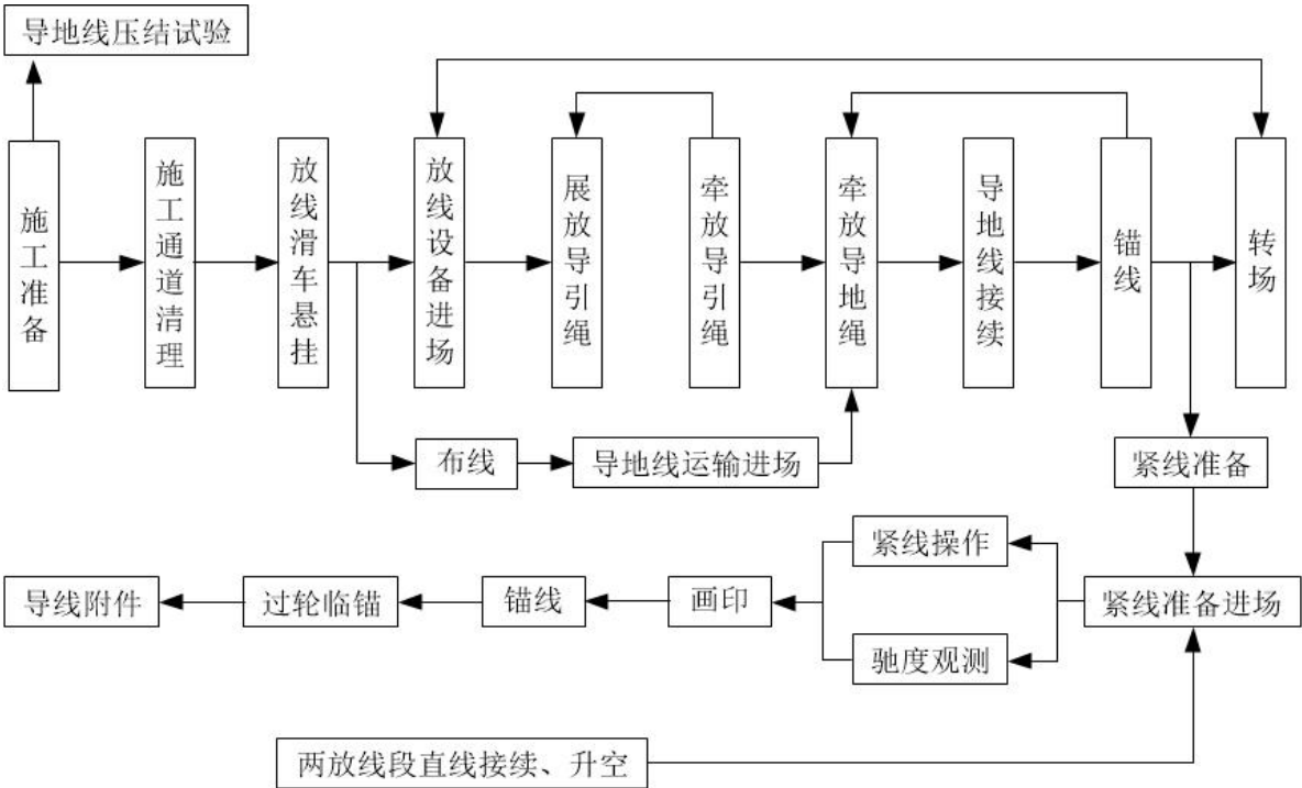
图 3.1-4 架线施工工艺流程图
