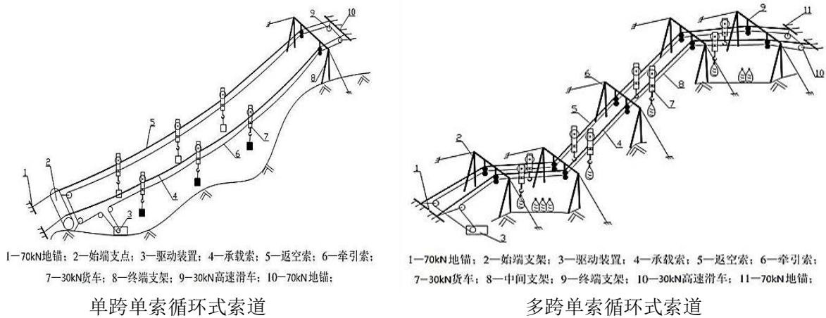
图 3.1-5 索道示意图
