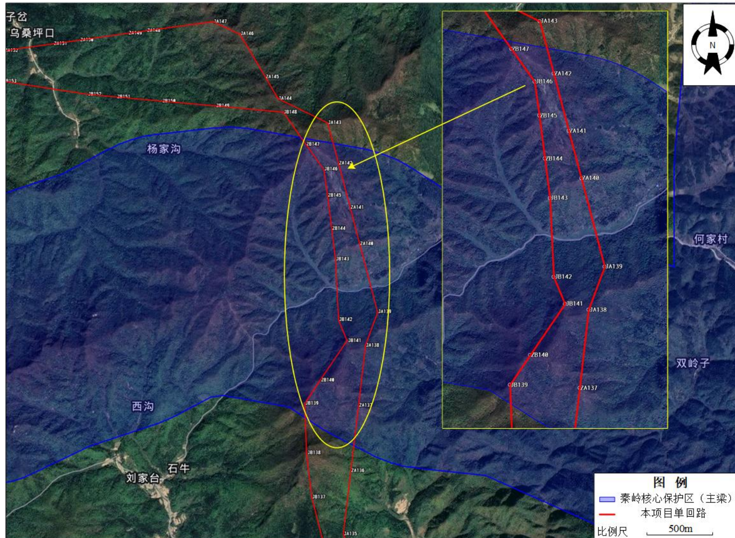
图 3.2-10 本项目输电线路穿越秦岭核心保护区（主梁）段相对位置关系示意图
