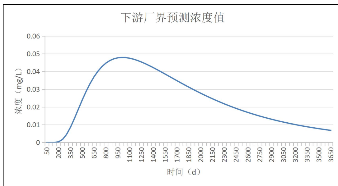
图 5.2.3-8 非正常泄漏后下游厂界石油类浓度图
