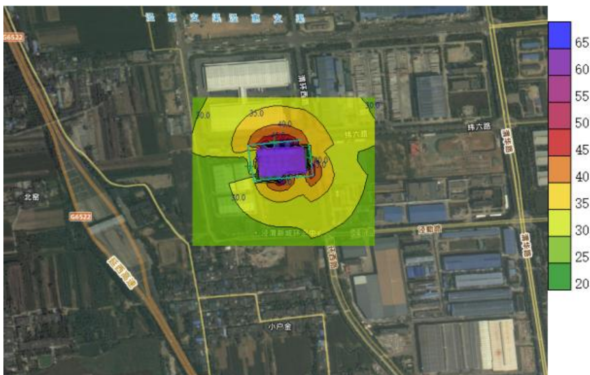
图 5.2.3-2 夜间贡献值等声级线图
