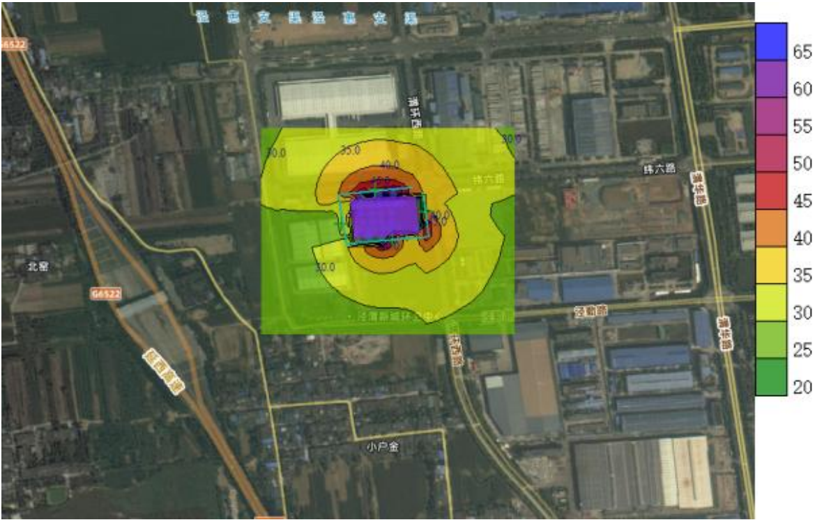
图 5.2.3-1 昼间贡献值等声级线图
