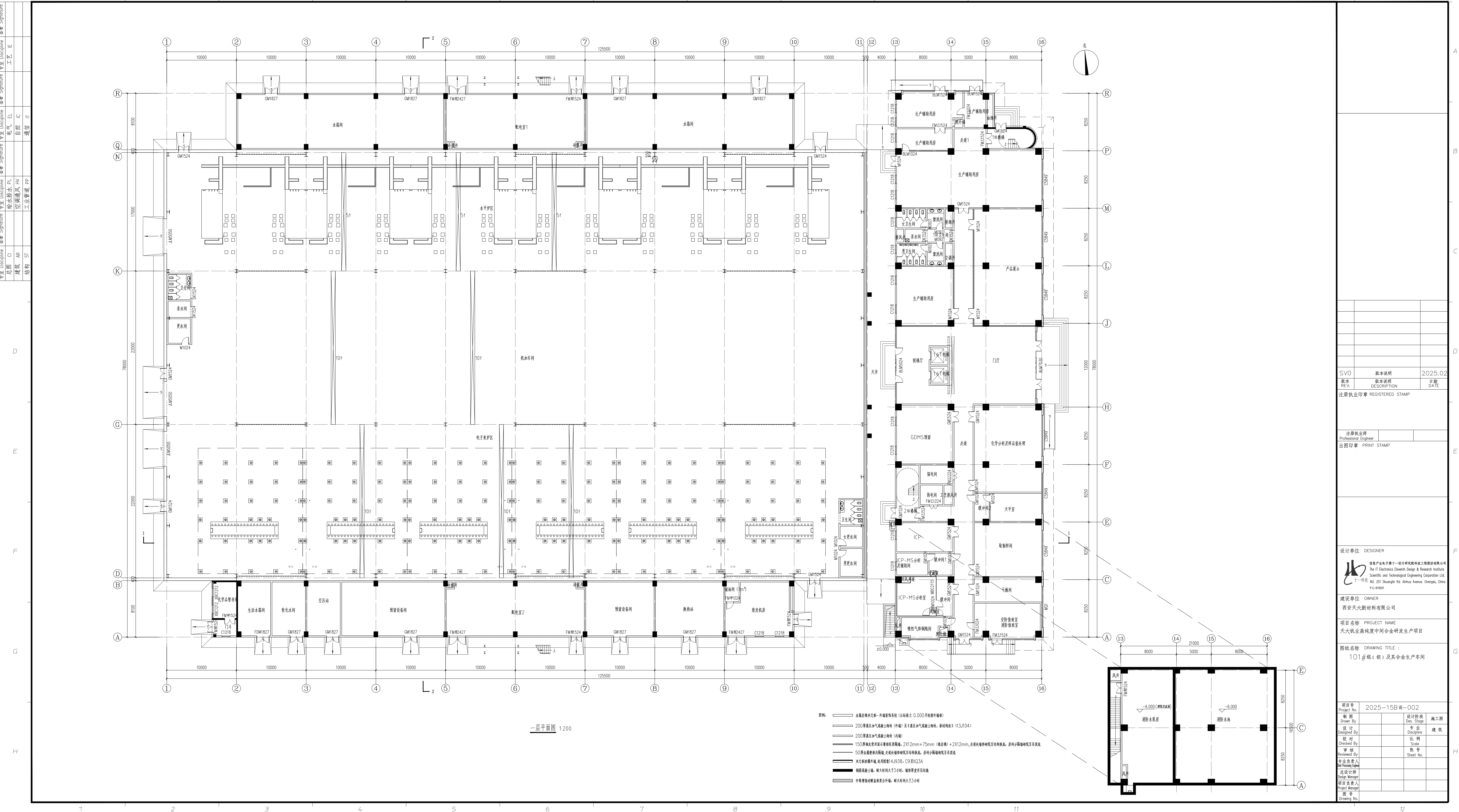
附图3-2 辅助车间（办公楼）1-5层平面布置图
