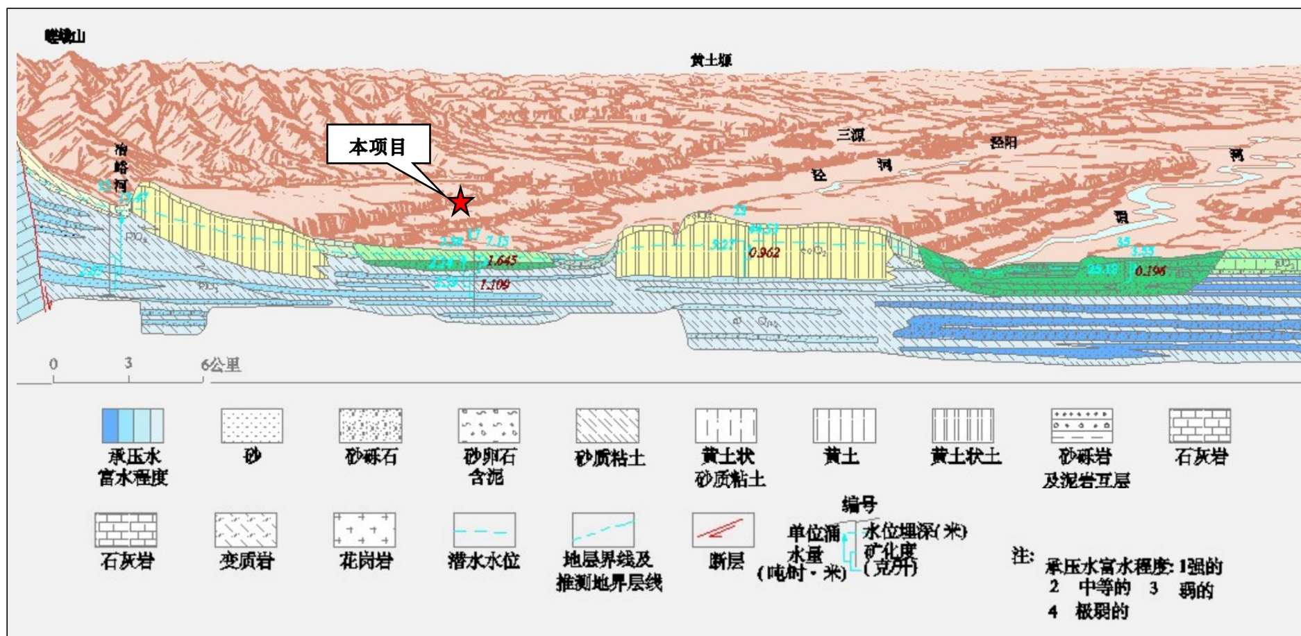
图 5.2.3-4 水文地质剖面图
