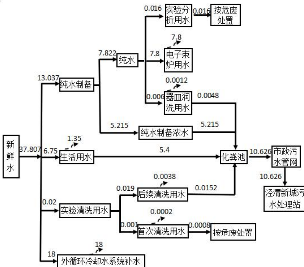
图 2.3.1-1 项目水平衡图 单位: \text{m}^3/\text{d}
