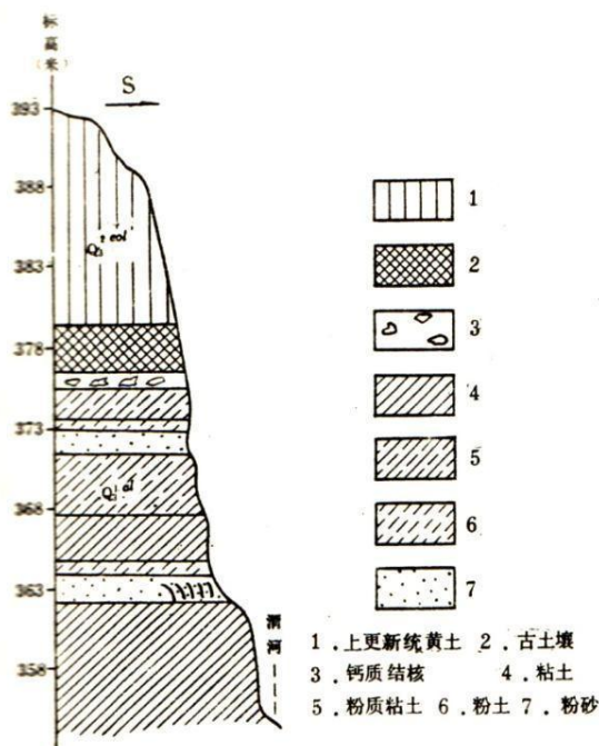
图 5.2.3-2 区域典型地层剖面图
