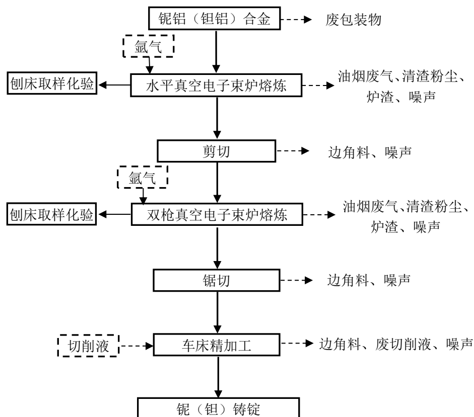
图 3.1.2-1 铌（钽）铸锭生产工艺流程及产污环节图
