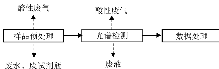
图 3.1.2-3 实验检测工艺流程及产污环节图
