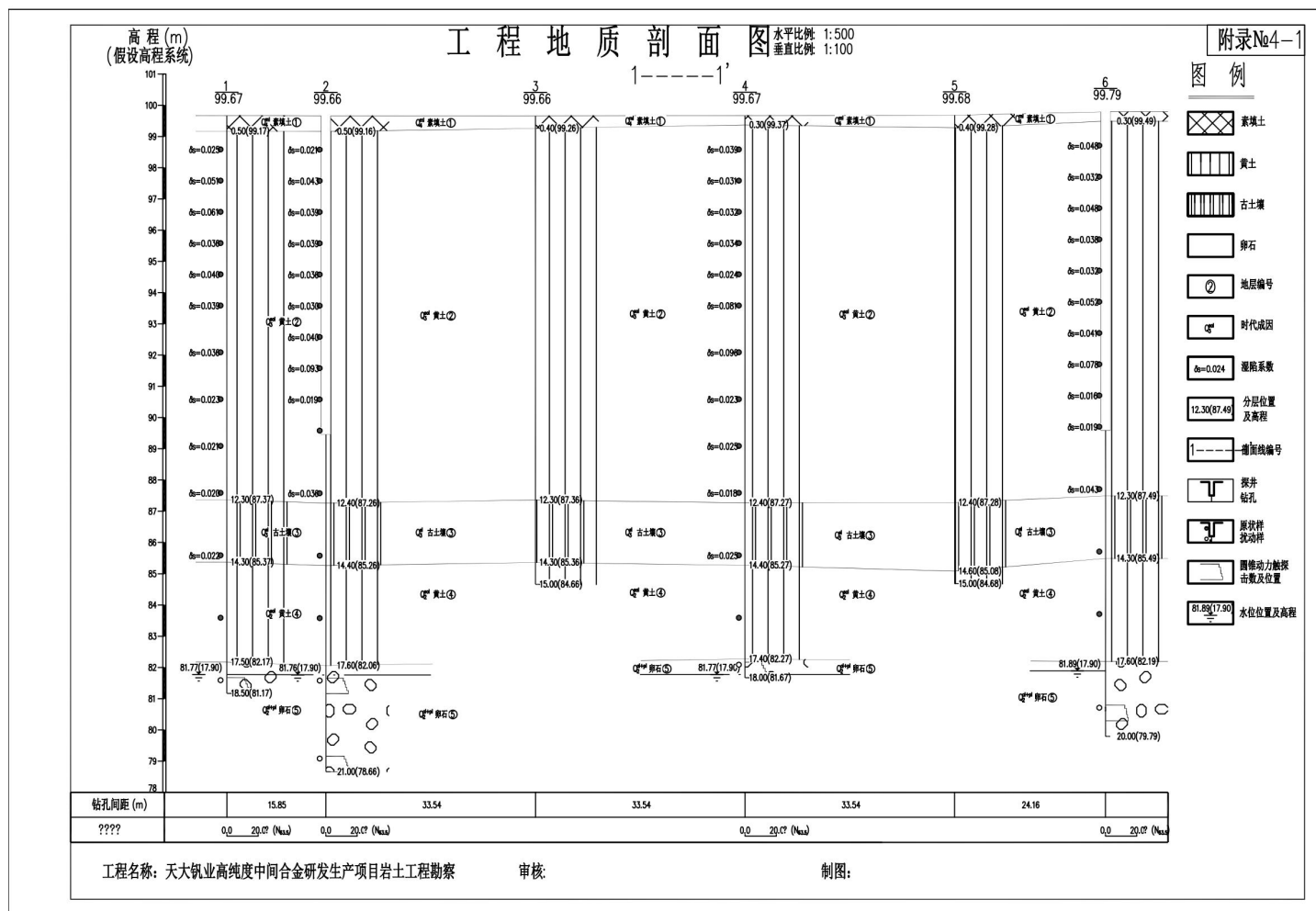
图 5.2.3-5 项目场地工程地质剖面图
