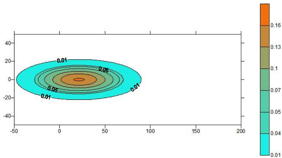
非正常泄漏 365d 石油类污染物浓度图
