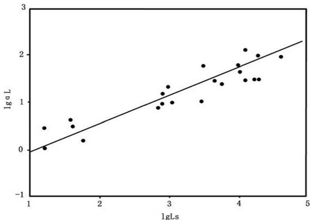
图 5.2.3-6 孔隙介质数值模型的 \lg \alpha_L - \lg L_s 图
