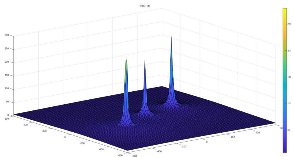
图 6.1-6 (b) 工作模式 3 电场强度预测结果等值线图 2 (单位: V/m)
