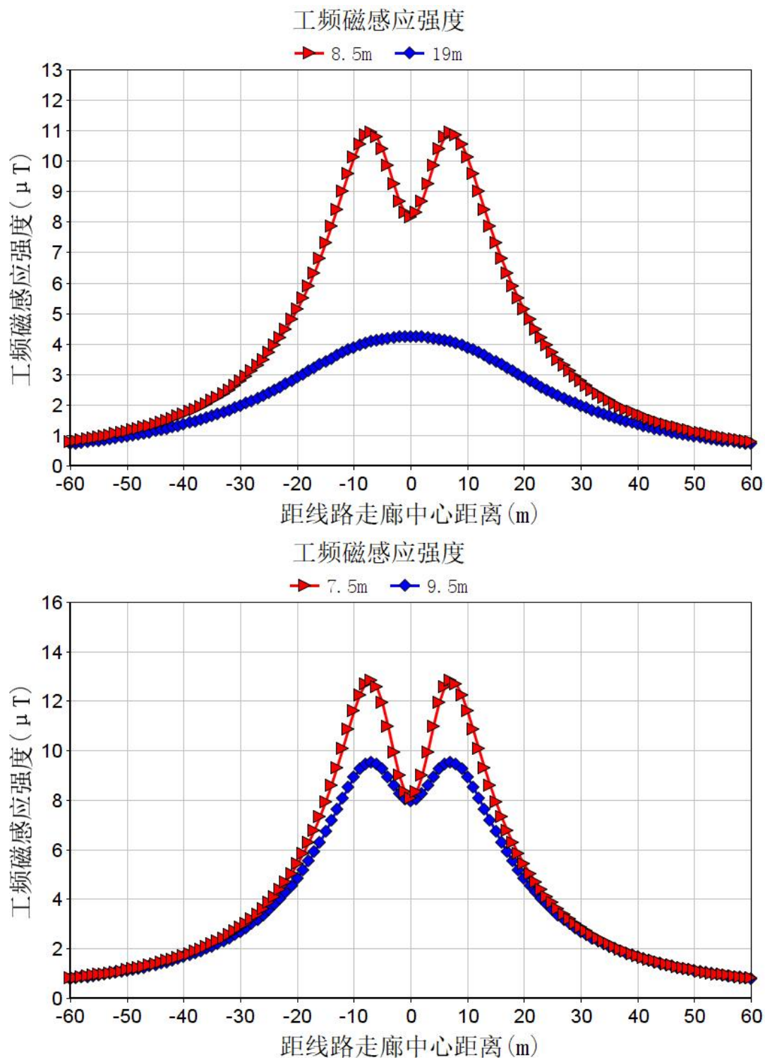
图 6.1-6 330kV 同塔双回输电线路工频磁感应强度分布图
