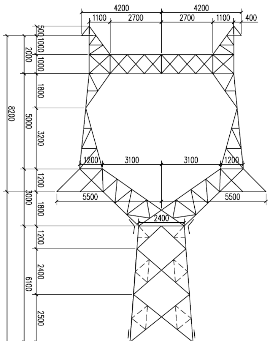
图 7.1-2 预测塔型图
