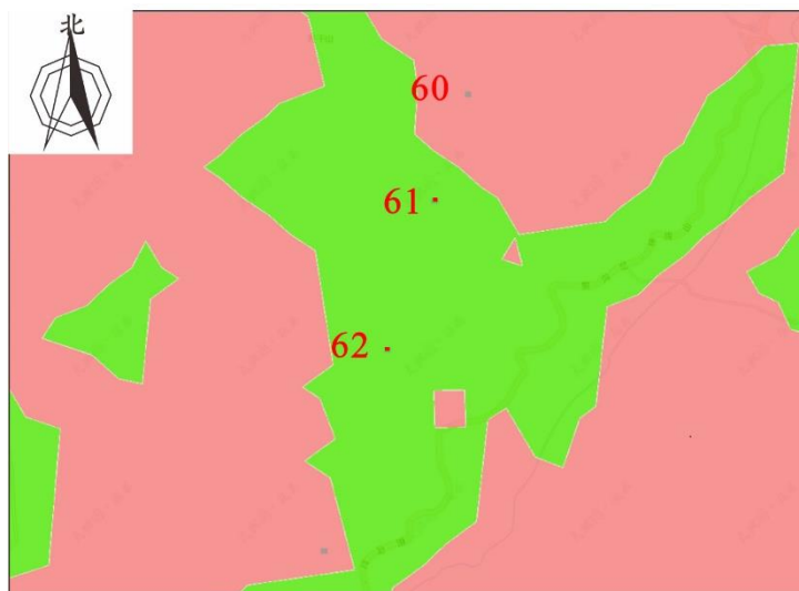
图 1-8 工程杆塔 60 号~61 号与陕西省“三线一单”分区管控单元位置及线路走向图
