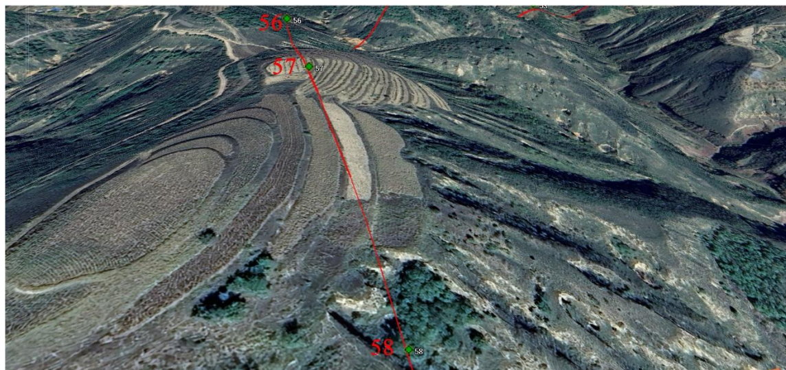
图 1-7 工程杆塔 56 号~58 号与陕西省“三线一单”分区管控单元位置及线路走向图
