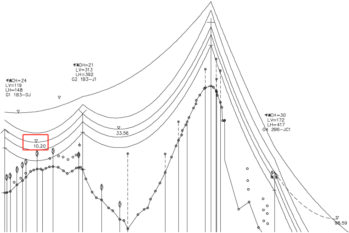
图 7.1-1 线路局部平断面图
