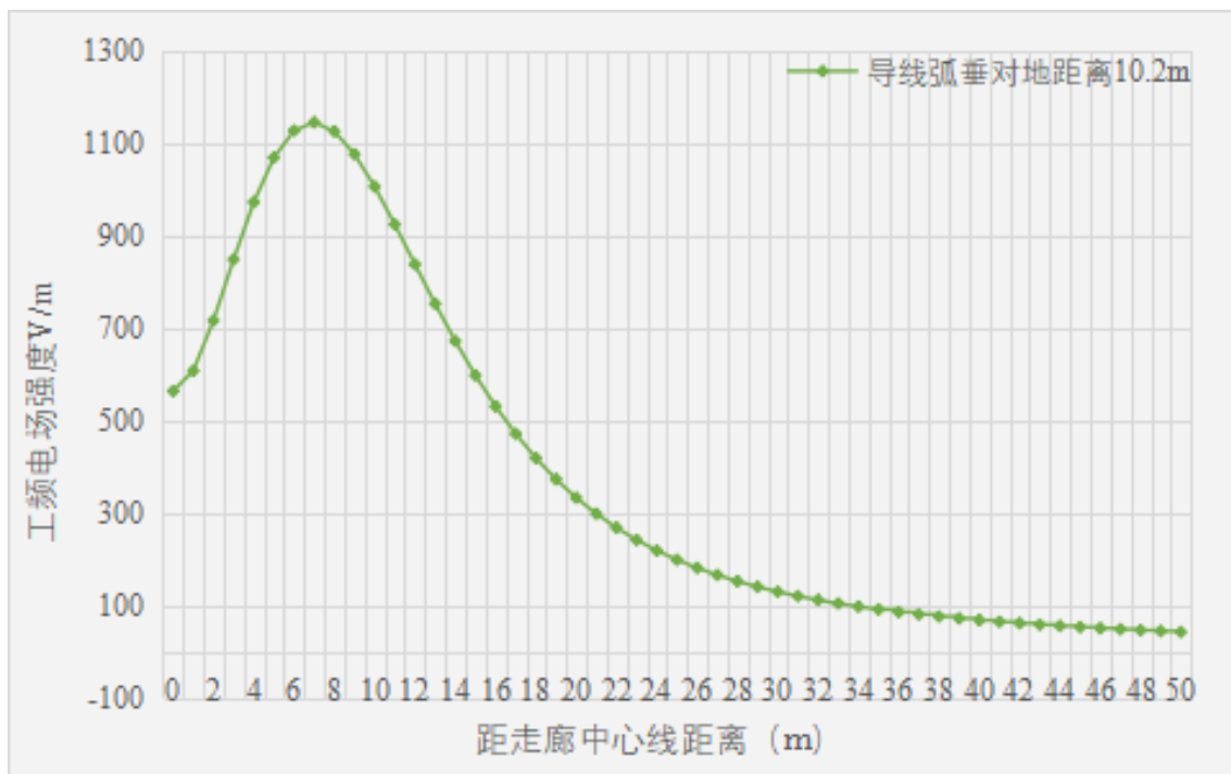
图 7.1-3 2B6-ZMCK 型塔工频电场强度趋势图
