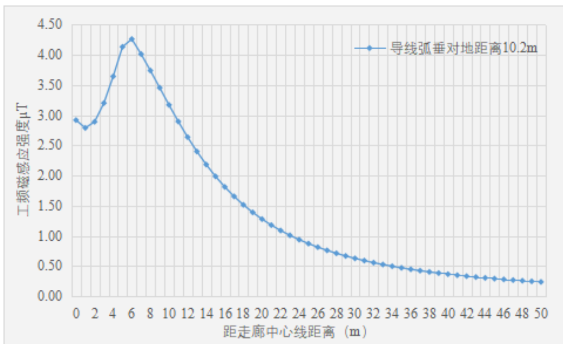
图 7.1-4 2B6-ZMCK 型塔工频磁感应强度趋势图
