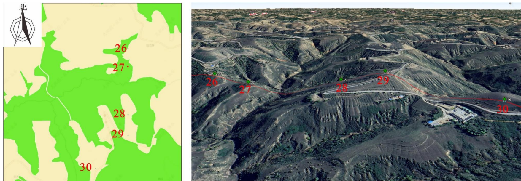
图 1-4 工程杆塔 26 号~30 号与陕西省“三线一单”分区管控单元位置及线路走向图
