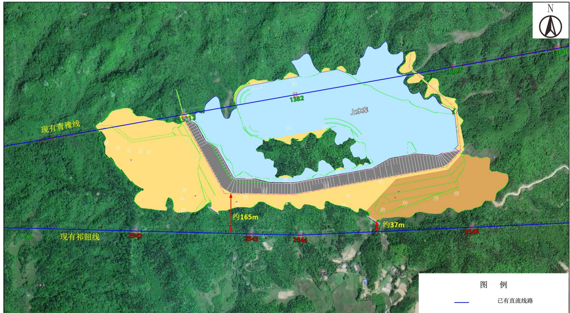
图1.1-2 优化后上水库与特高压线路位置关系示意图
