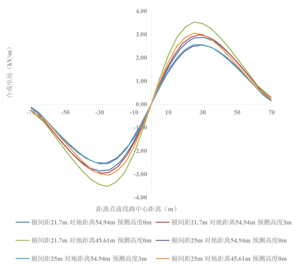
图 6.1-3 祁韶线迁改段直流线路地面合成电场强度预测结果
