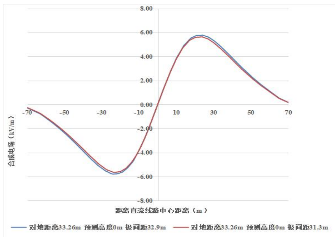
图 6.1-2 青豫线迁改段直流线路地面合成电场强度预测结果
