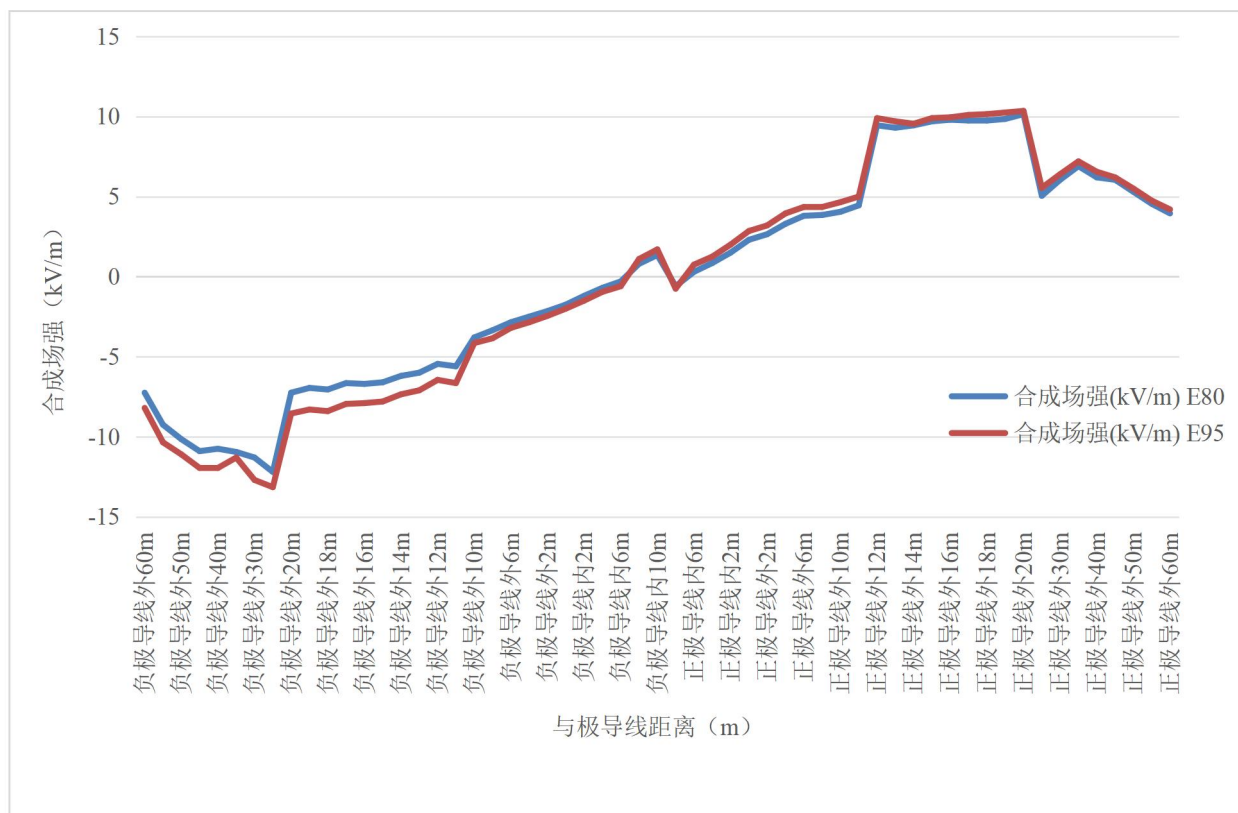
图 6.1-1 已有青豫线甘肃段衰减断面监测趋势线图
