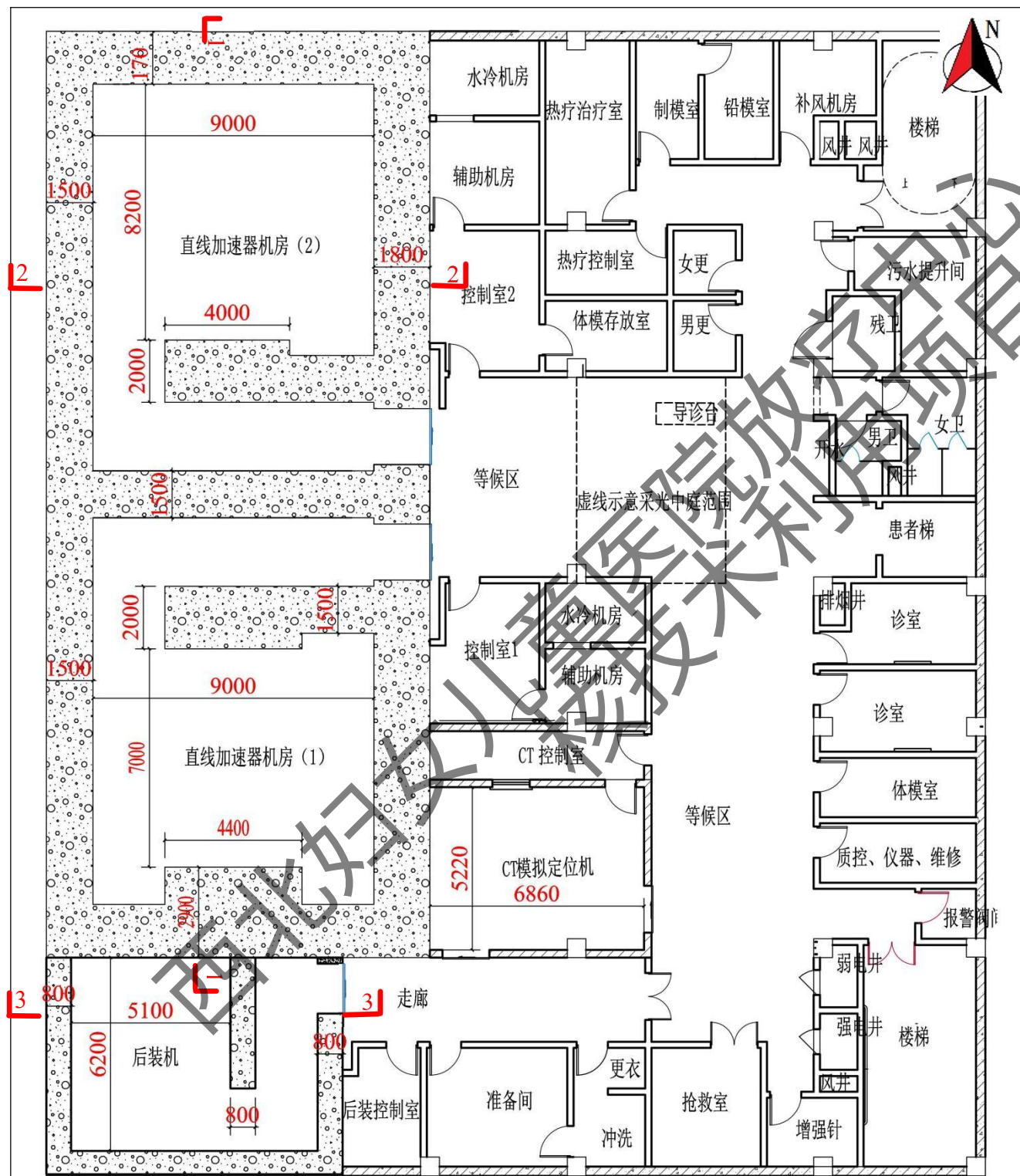
图 10-2 机房屏蔽示意图 (单位: mm)
