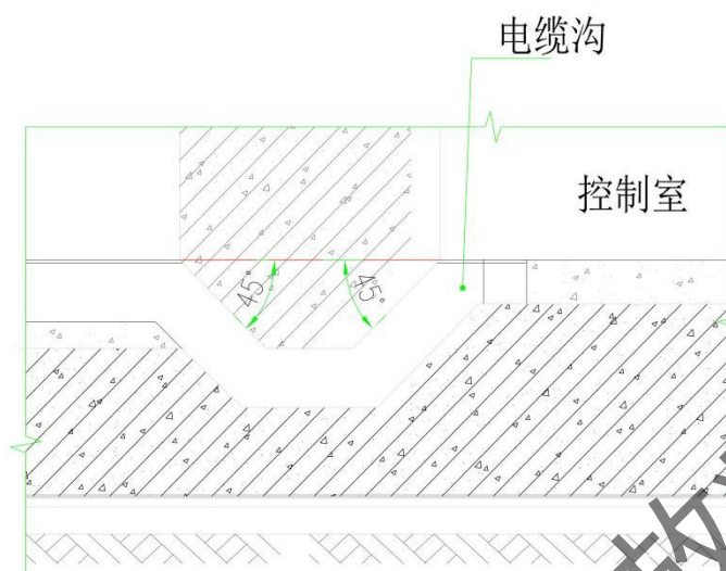
图 10-7 电缆沟穿屏蔽墙设计图
