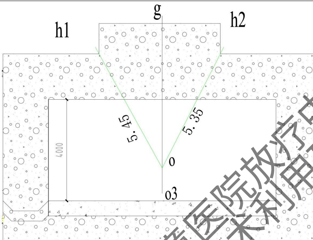
图 11-4 直线加速器机房关注点设定示意图（剖面 1-1）
