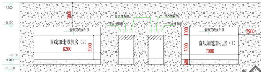
图 10-3 加速器机房屏蔽示意剖面图（剖面 1-1）（单位：mm）
