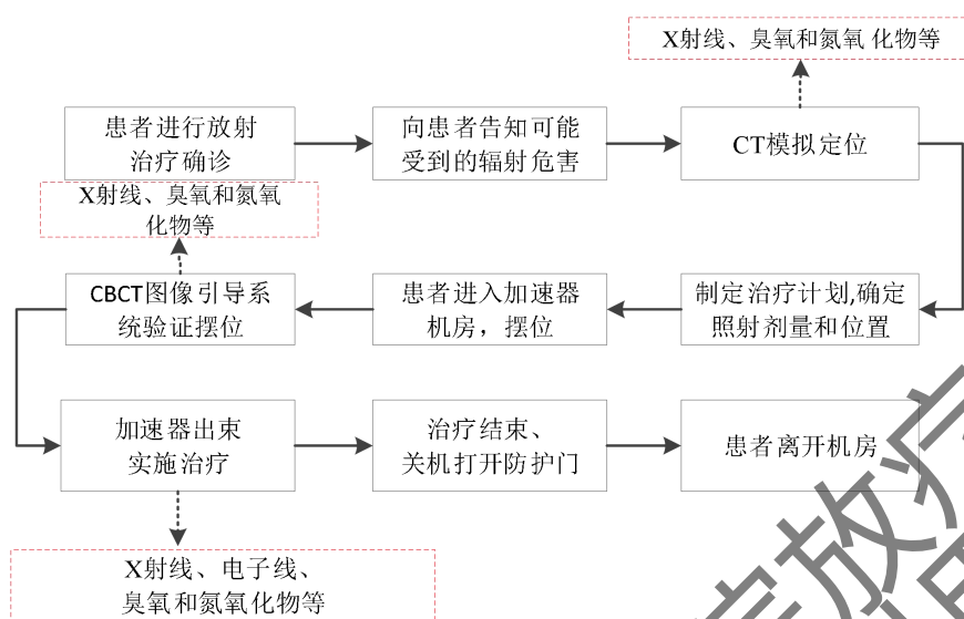
图 9-3 电子直线加速器治疗流程及产污环节示意图
