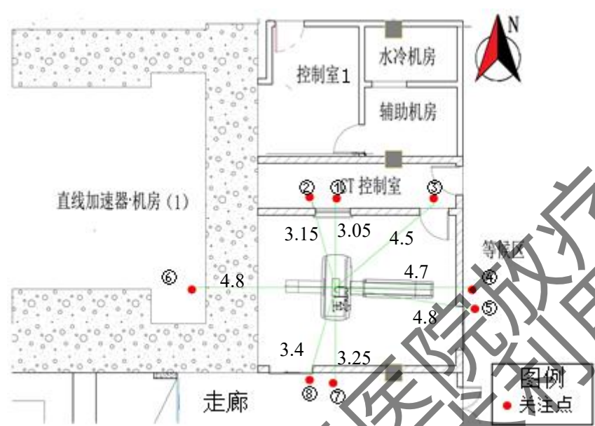
图 11-8 CT 模拟定位机房关注点示意图（平面）（单位：m）
