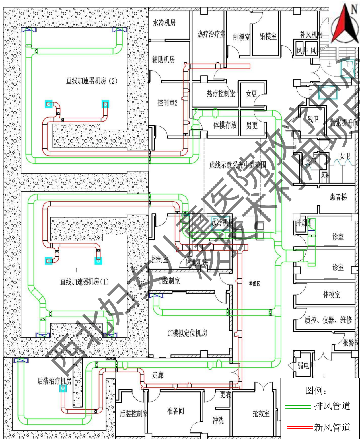
图 10-8 通风管道平面图
