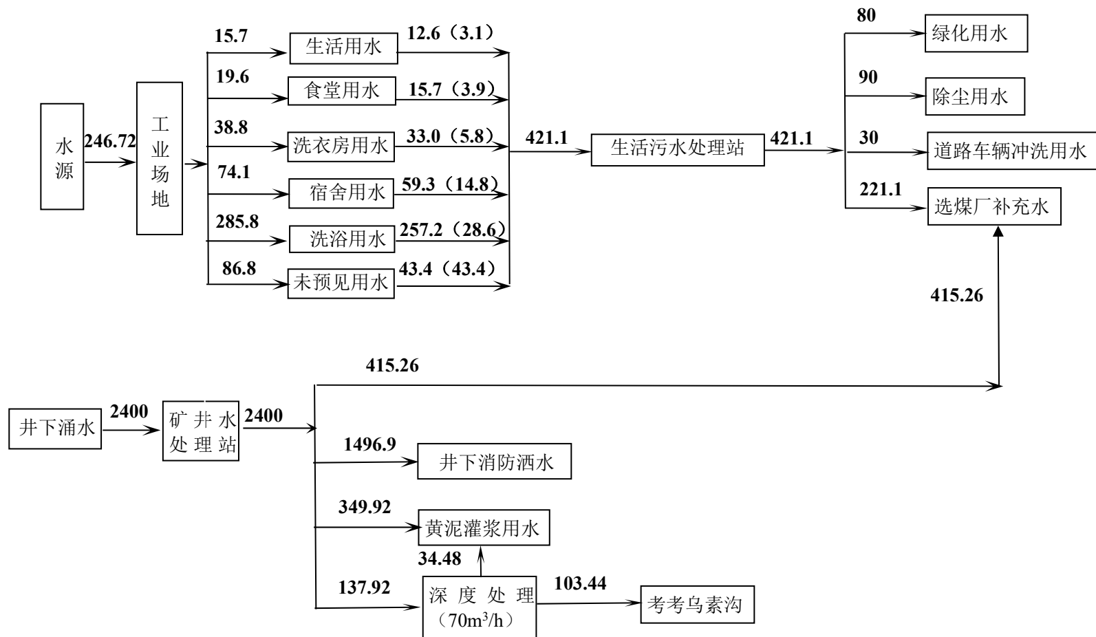
图 2.3.2-3 四门沟煤矿非采暖期用水平衡图
