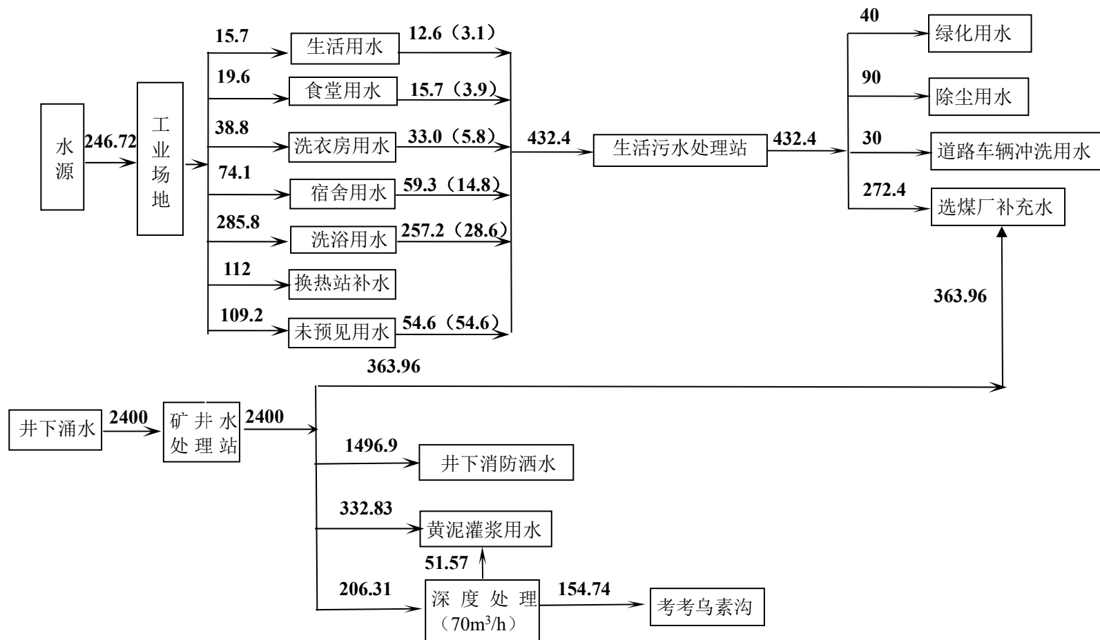
图 2.3.2-2 四门沟煤矿采暖期用水平衡图
