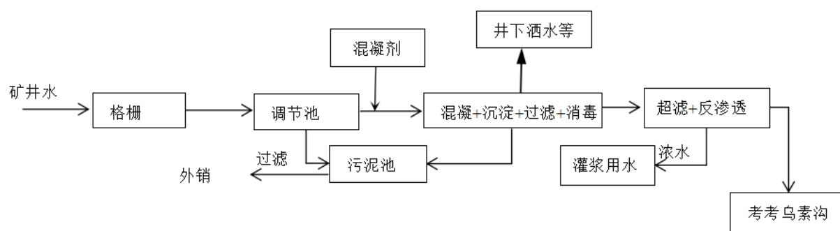
图 2.2.9-2 矿井水处理工艺流程图
