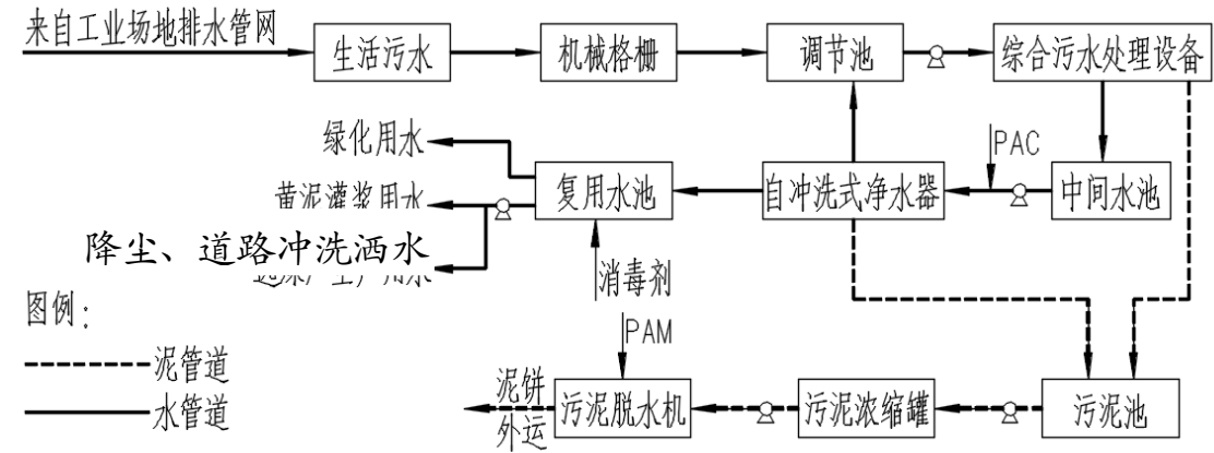
图 2.2.9-1 生活污水处理工艺流程图
