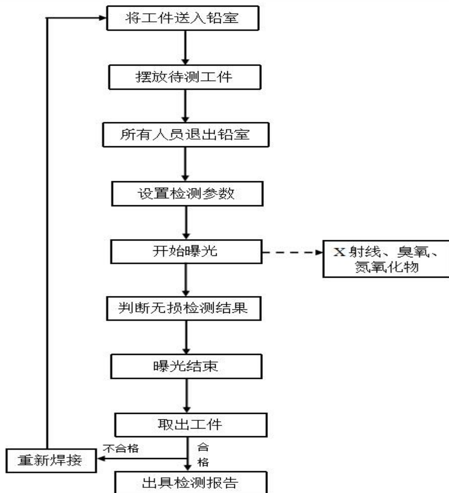
图 9-1 检测工艺流程图及产污环节图
