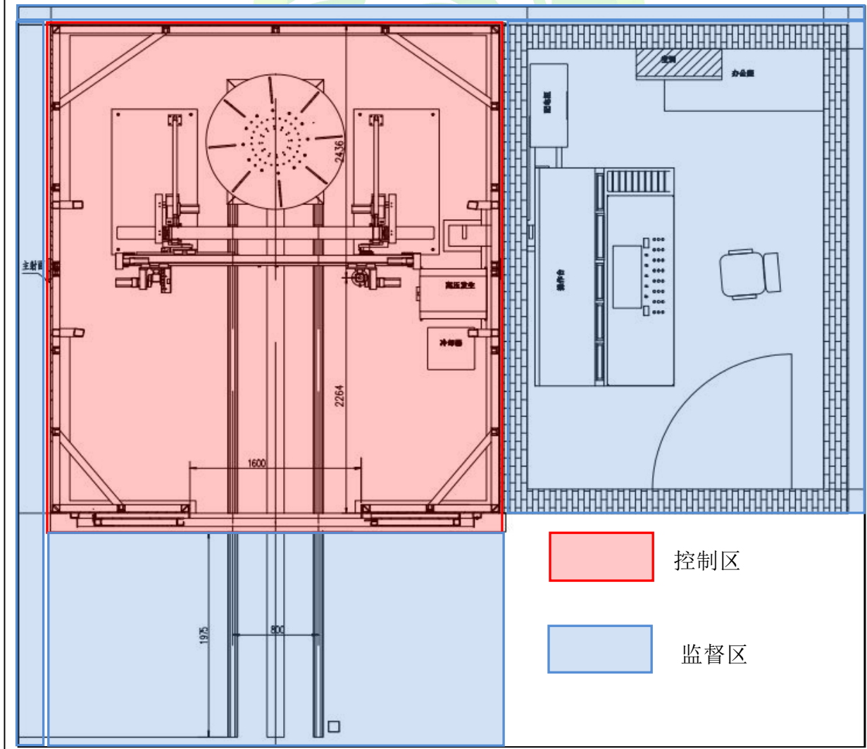
图 10-1 辐射工作场所分区图
