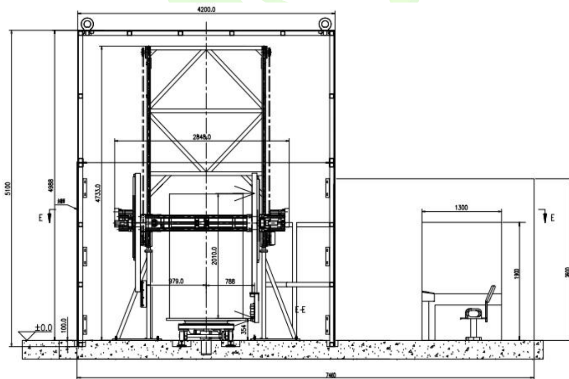
图 10-3 铅房剖面图
