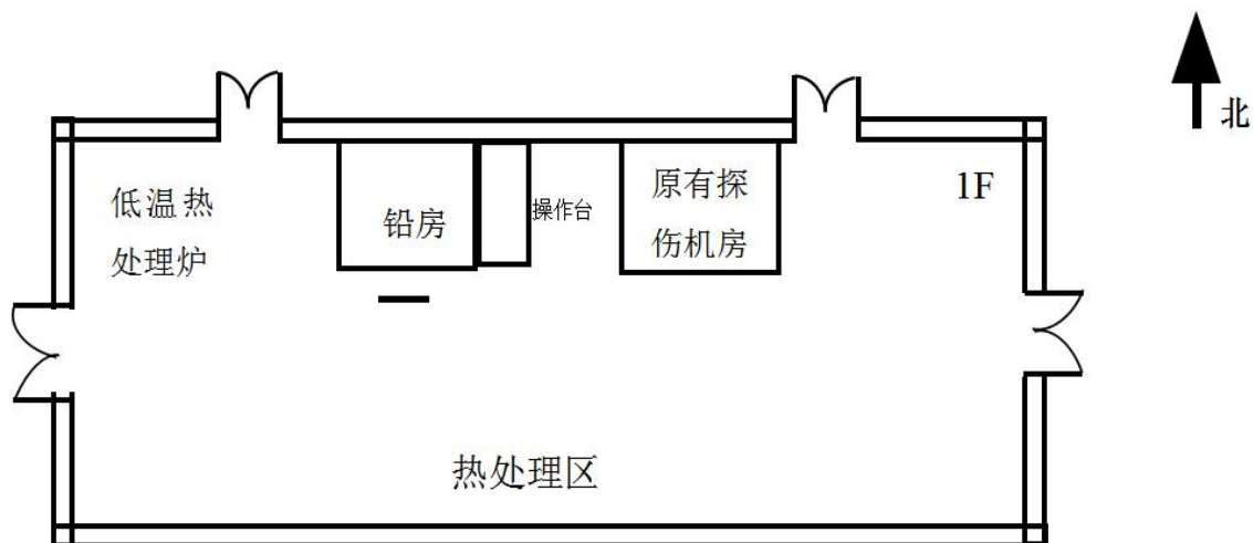
图 10-2 铅房平面布置图
