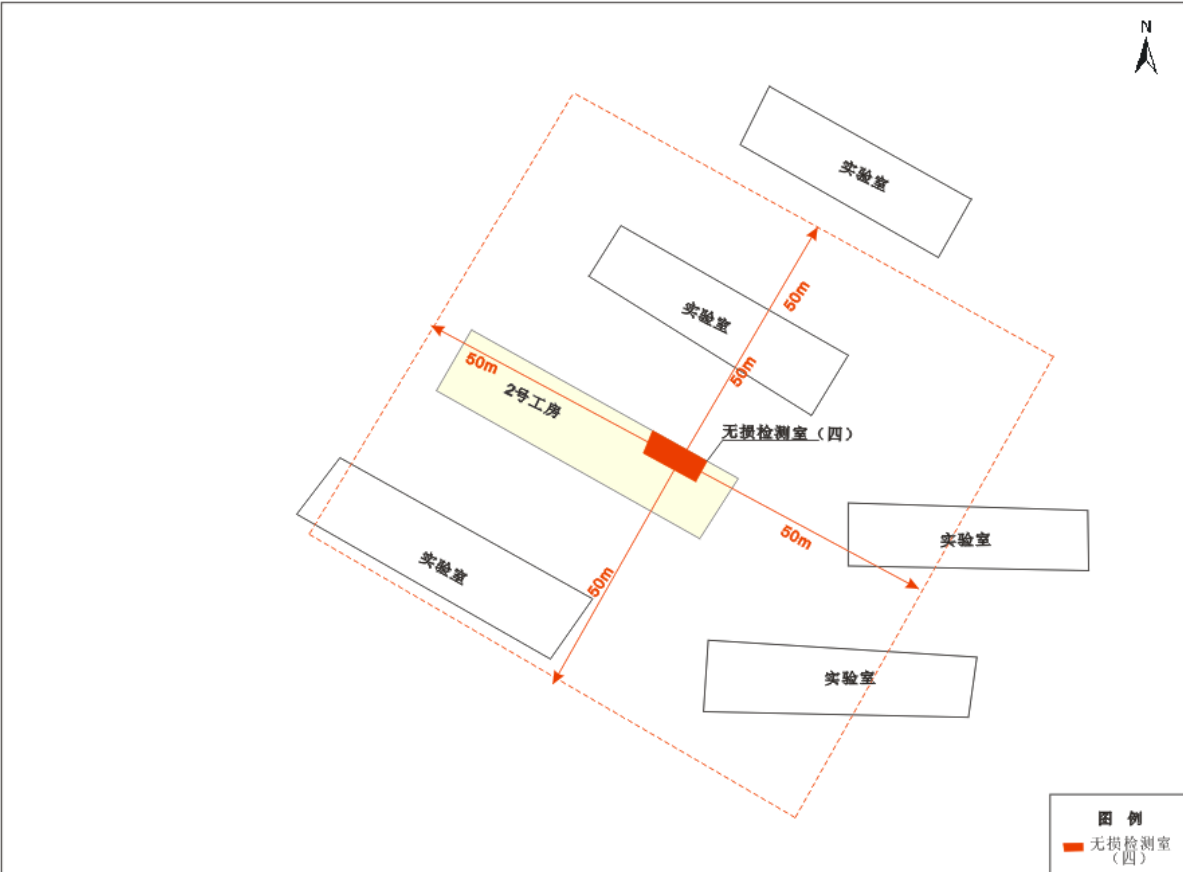
图 1-7 无损检测室（四）周边环境关系示意图
