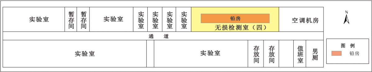
图 1-8 无损检测室（四）平面布置图
