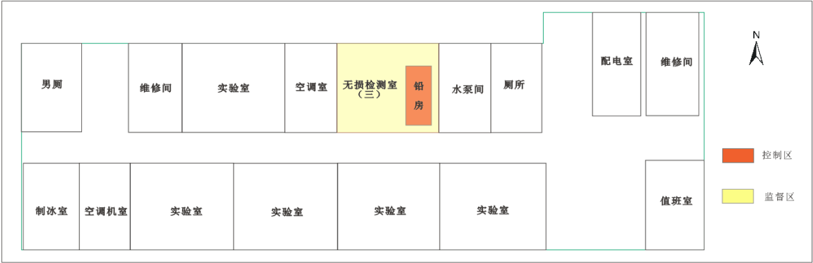
图 10-3 无损检测室（三）辐射工作场所分区示意图
