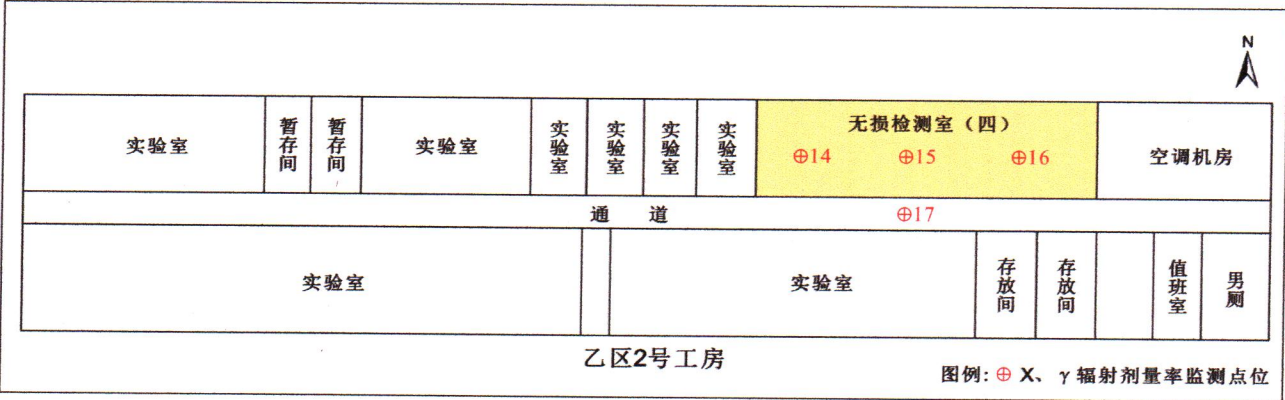
图3-3 乙区2号工房监测点位示意图
