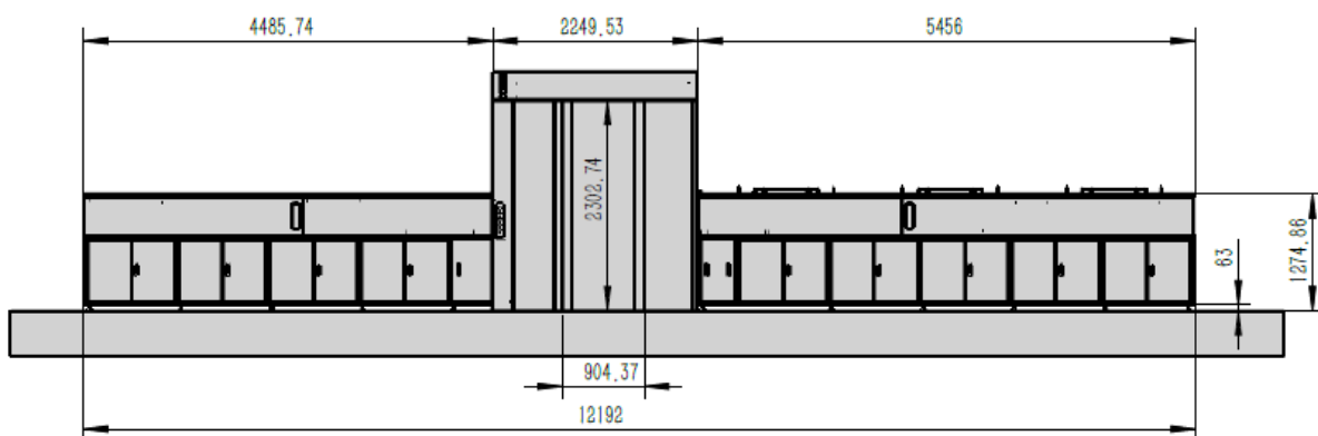
图 10-13 无损检测室（四）立面图
