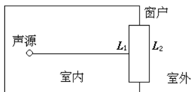
图 5.2-15 室内声源向室外传播示意图
