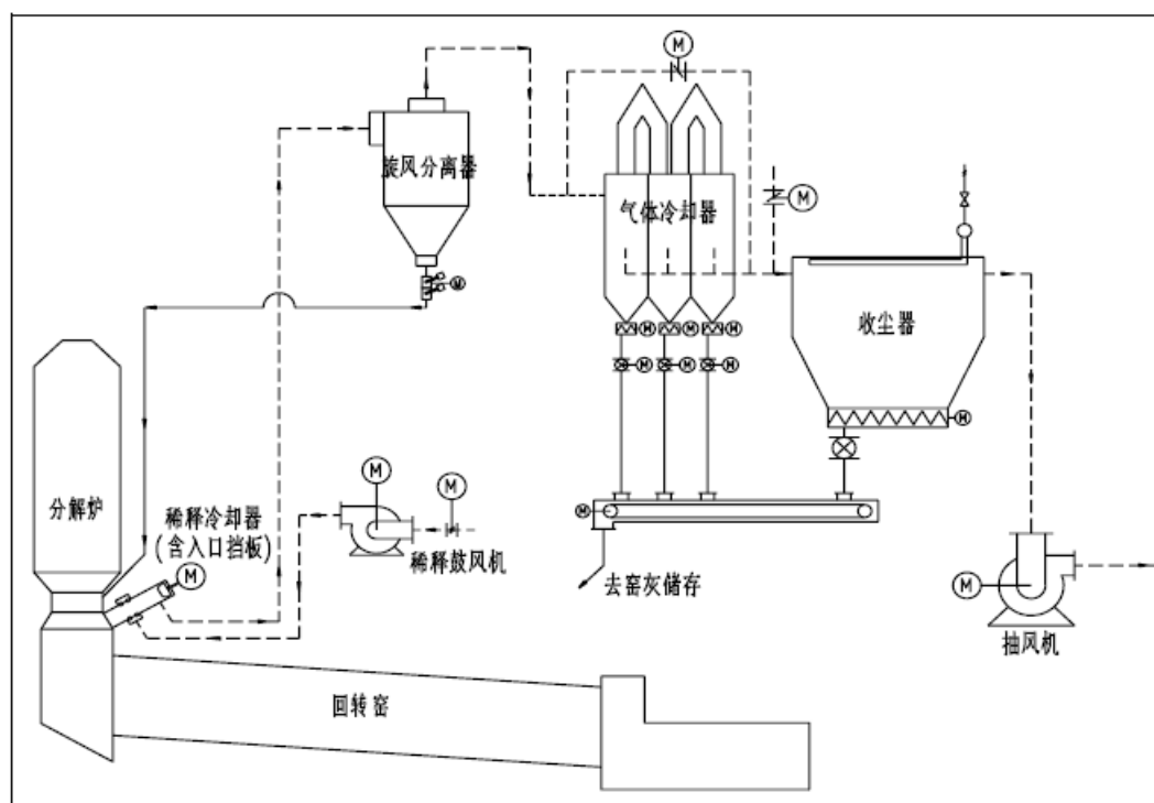
图 3.2-3 旁路放风工艺流程图
