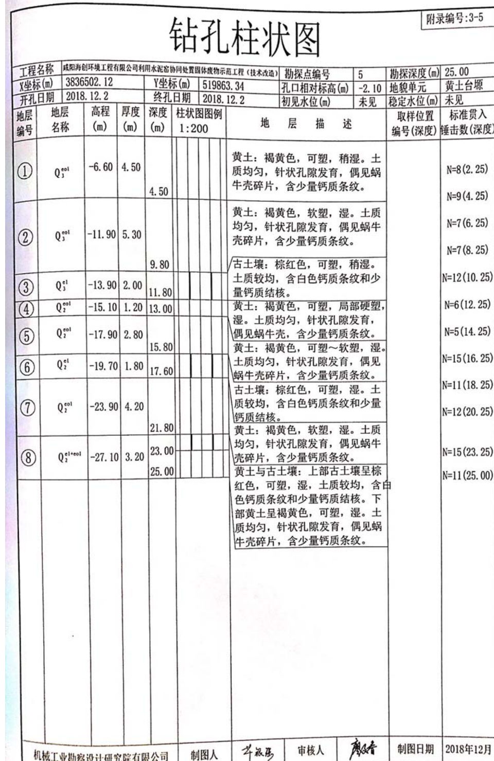
图 5.2-14 钻孔柱状图
