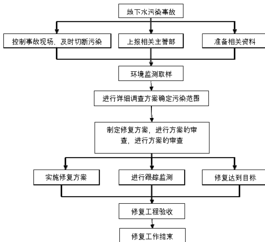
图 6.3-3 地下水污染应急治理程序框图
