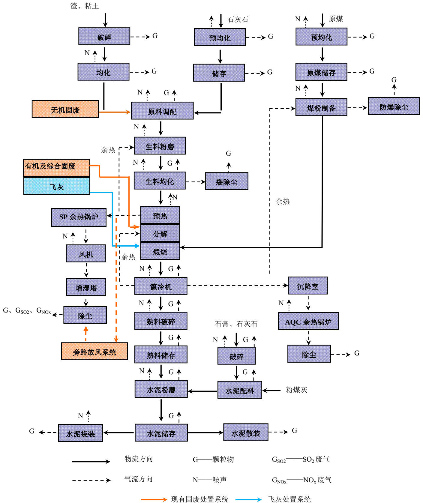
图 3.2-2 协同处置固废后水泥生产线工艺流程及产污环节图
